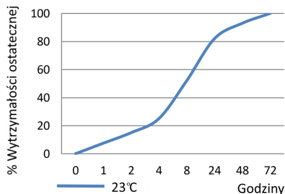
Wykres przyrostu wytrzymałości
