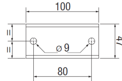
Wspornik skrzydło
