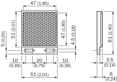
Rysunek wymiarowy (Wymiary w mm)
