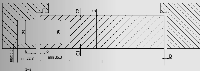
Wymiary gniazda
