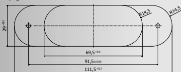
Wymiary gniazda
