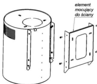
Rys. 8 Montaż okapu (w wersji przyściennej)
