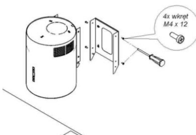
Rys. 8 Montaż okapu (w wersji przyściennej)
