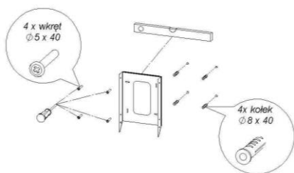
Rys. 7 Montaż elementu mocującego
