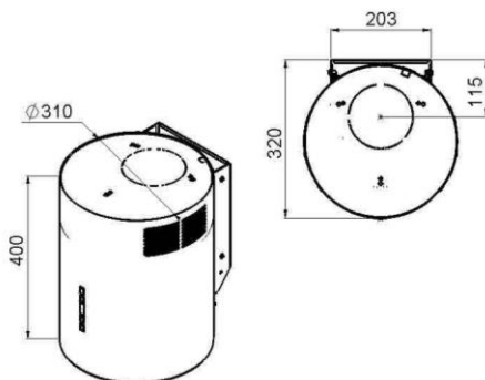
Rys. 2 Wymiary gabarytowe okapu
