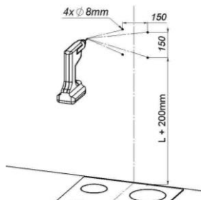
Rys. 7 Montaż elementu mocującego
