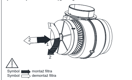
Rys. 12 Wymiana filtra węglowego.
