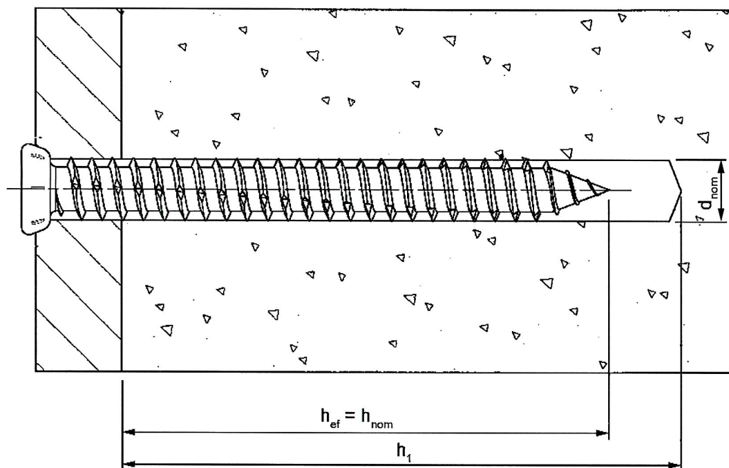
Rysunek B1. Parametry montażu wkrętów stalowych WHO
