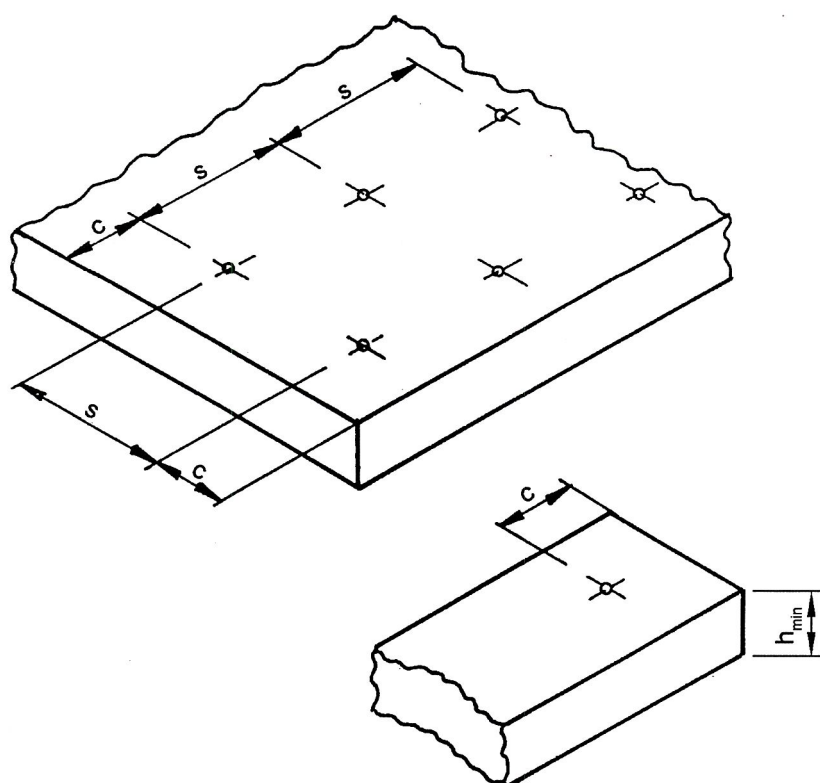
Rysunek B1. Parametry montażu wkrętów stalowych WHO
