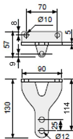
Uchwyt montażowy od strony silnika
