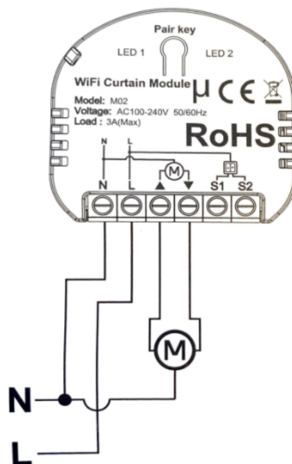
Podłączenie bez przełącznika
