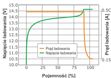
Charakterystyka ładowania
