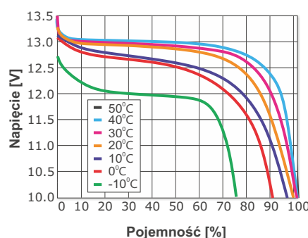
Charakterystyki rozładowania względem temperatury
