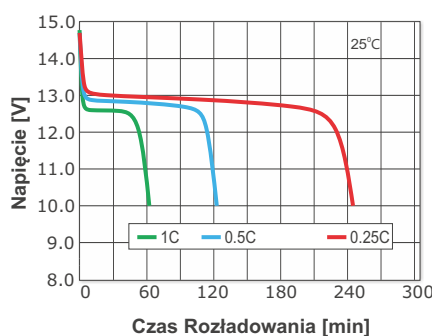
Charakterystyki rozładowania
