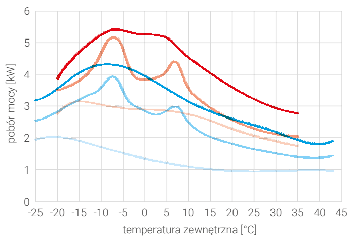
Charakterystyki poboru mocy - Prima 14GT
