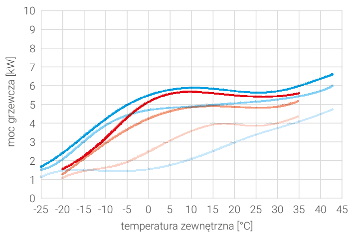
Charakterystyki mocy grzewczej - Prima 4GT
