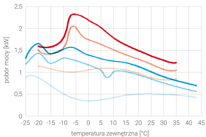
Charakterystyki poboru mocy - Prima 4GT
