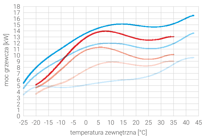
Charakterystyki mocy grzewczej - Prima 14GT
