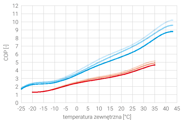
Charakterystyki COP - Prima 14GT COP 35 max COP 35 nor COP 35 min COP 55 max COP 55 nor COP 55 min
