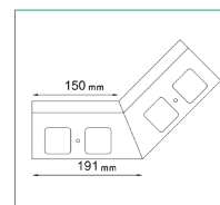
NAROŻNIK WEWNĘTRZNY K301 135
