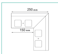
NAROŻNIK ZEWNĘTRZNY K301 90
