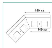
NAROŻNIK ZEWNĘTRZNY K301 135
