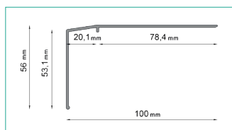
PROFIL OKAPOWY K301
