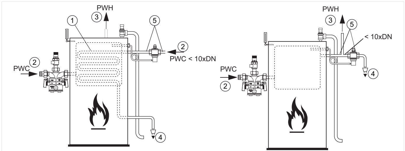
Rys. 1 Przykład standardowej instalacji zaworu zabezpieczenia odpływowego
