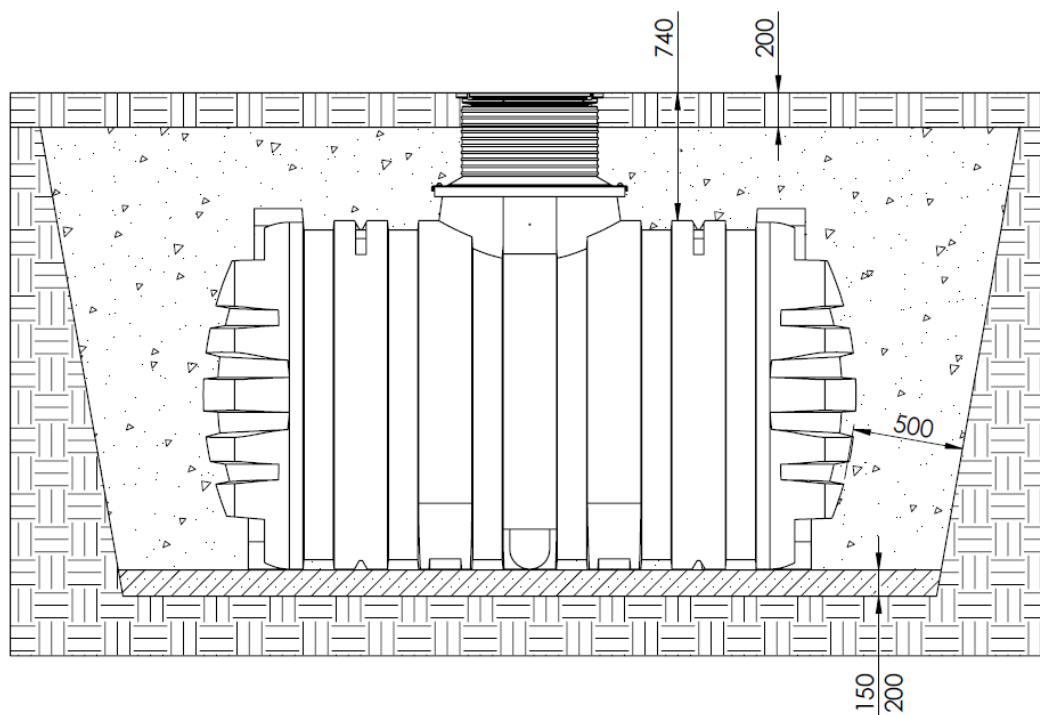
Rys.2 RainStore 10000/ RainStore Pro 10000 po montażu
