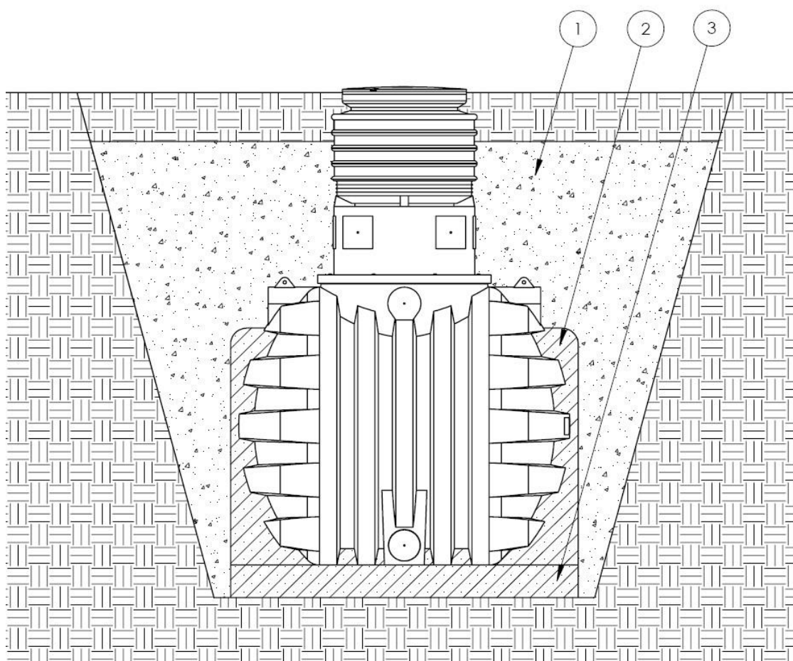
Rys.3 Zbiornik w otoczce z betonu
