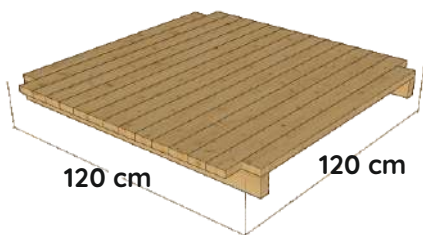
A-1 Ilość 1 szt.
