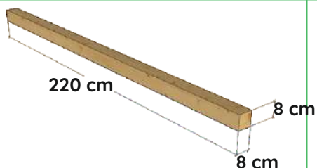
A-5 Ilość 4 szt.
