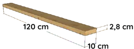
A-4 Ilość 2 szt.
