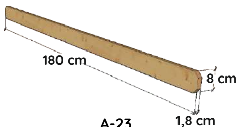
A-23 Ilość 2 szt.
