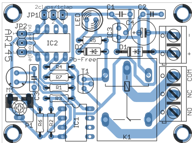
Rys. 1 Schemat montażowy
