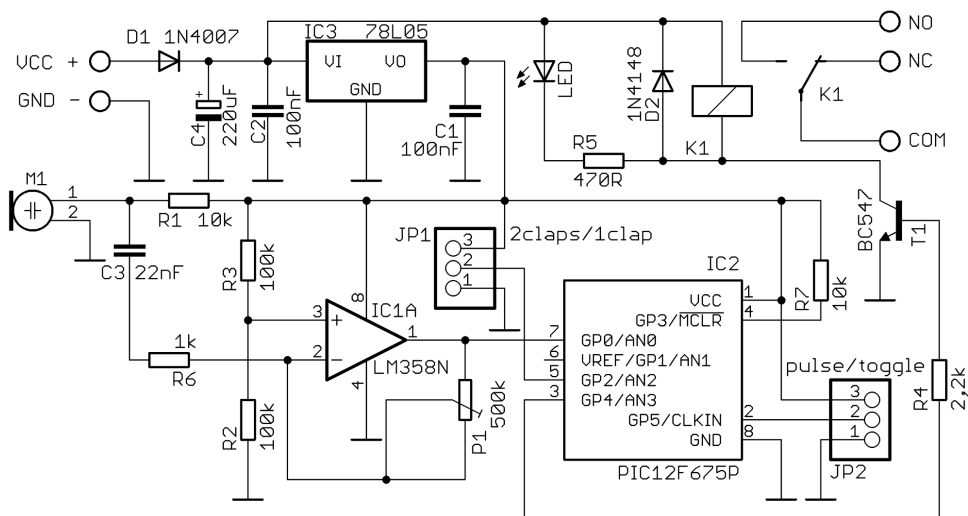
Rys. 2 Schemat ideowy
