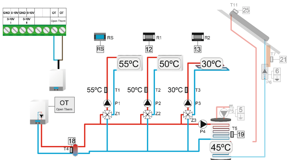
Przykład instalacji obsługiwanej za pomocą protokołu Open Therm.
