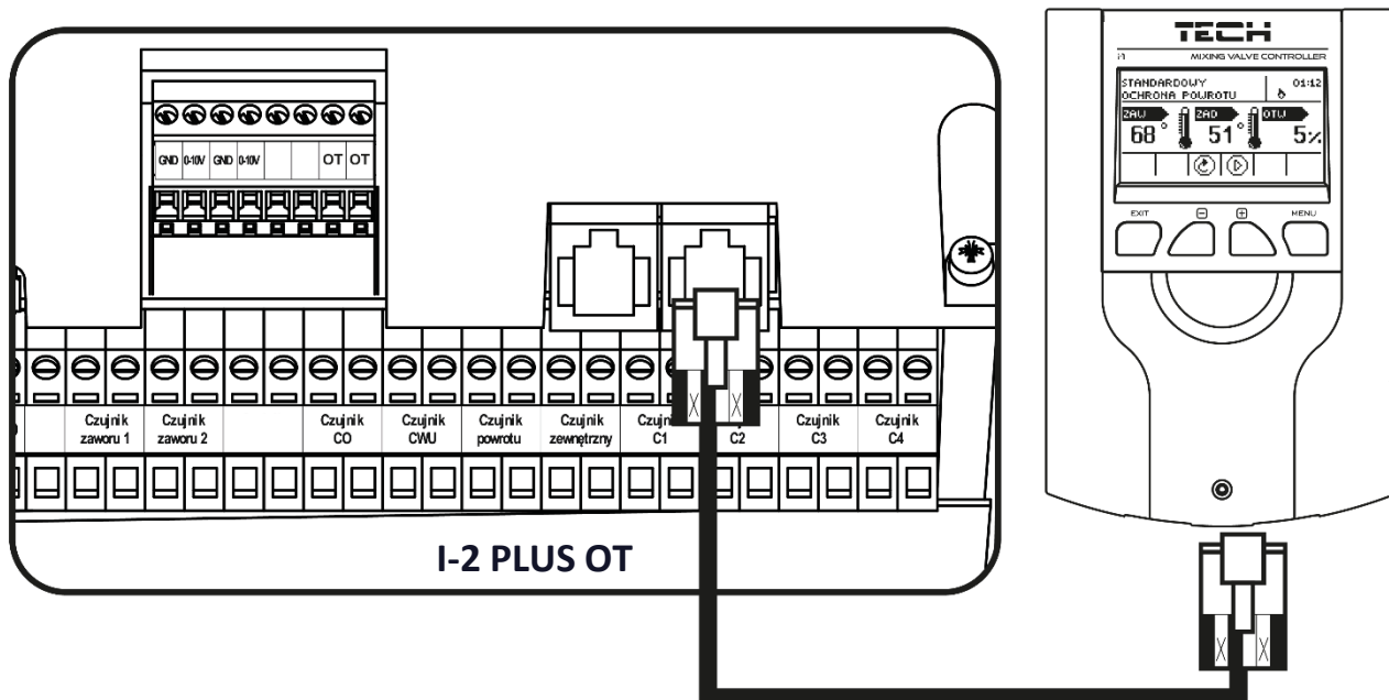
Przykładowe podłączenie zaworu dodatkowego ze sterownikiem głównym i-2 Plus OT
