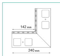
NAROŻNIK WEWNĘTRZNY K35 90
