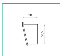
ODBOJNIKI PRZYŚCIENNE OPK35/OPK35B P+L
