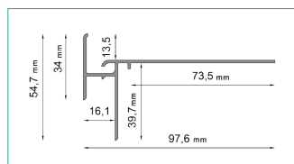
PROFIL OKAPOWY K35
