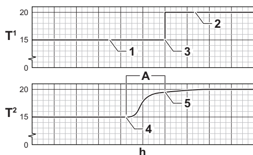
Rys.64 Wyprzedzające podwyższanie temperatury w pomieszczeniach a program czasowy
