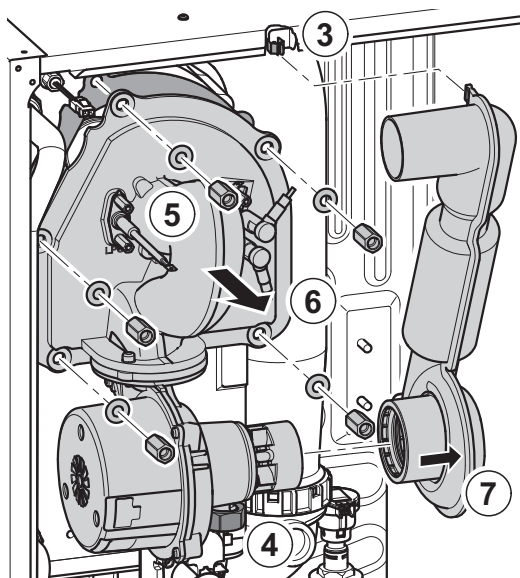
Rys.74 Wymontowywanie palnika gazowego
