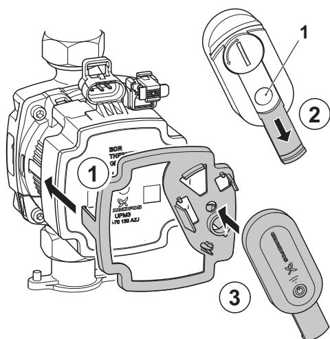
Rys.44 Montowanie czytnika ALPHA Reader
