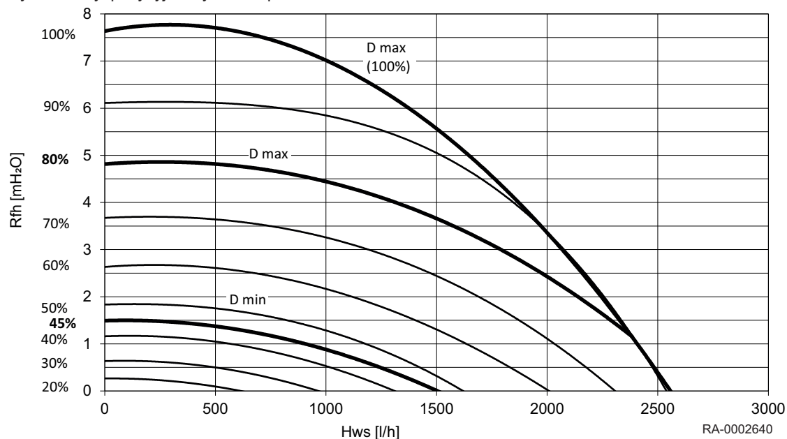
Rys.2 Dyspozycyjna wysokość podnoszenia WGB 28.2
