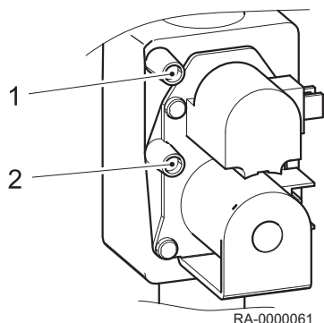
Rys.40 Zawór gazu WGB
