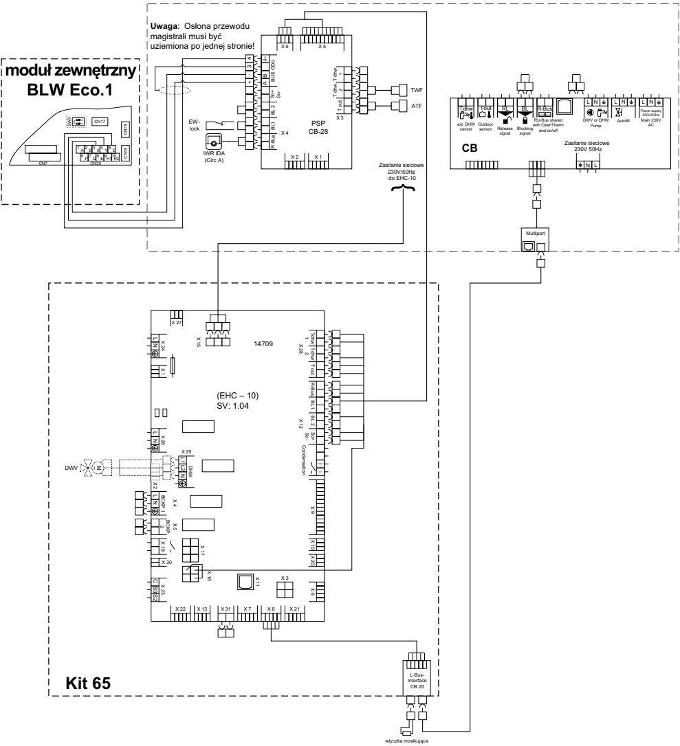
Rys.20 Schemat połączeń elektrycznych
