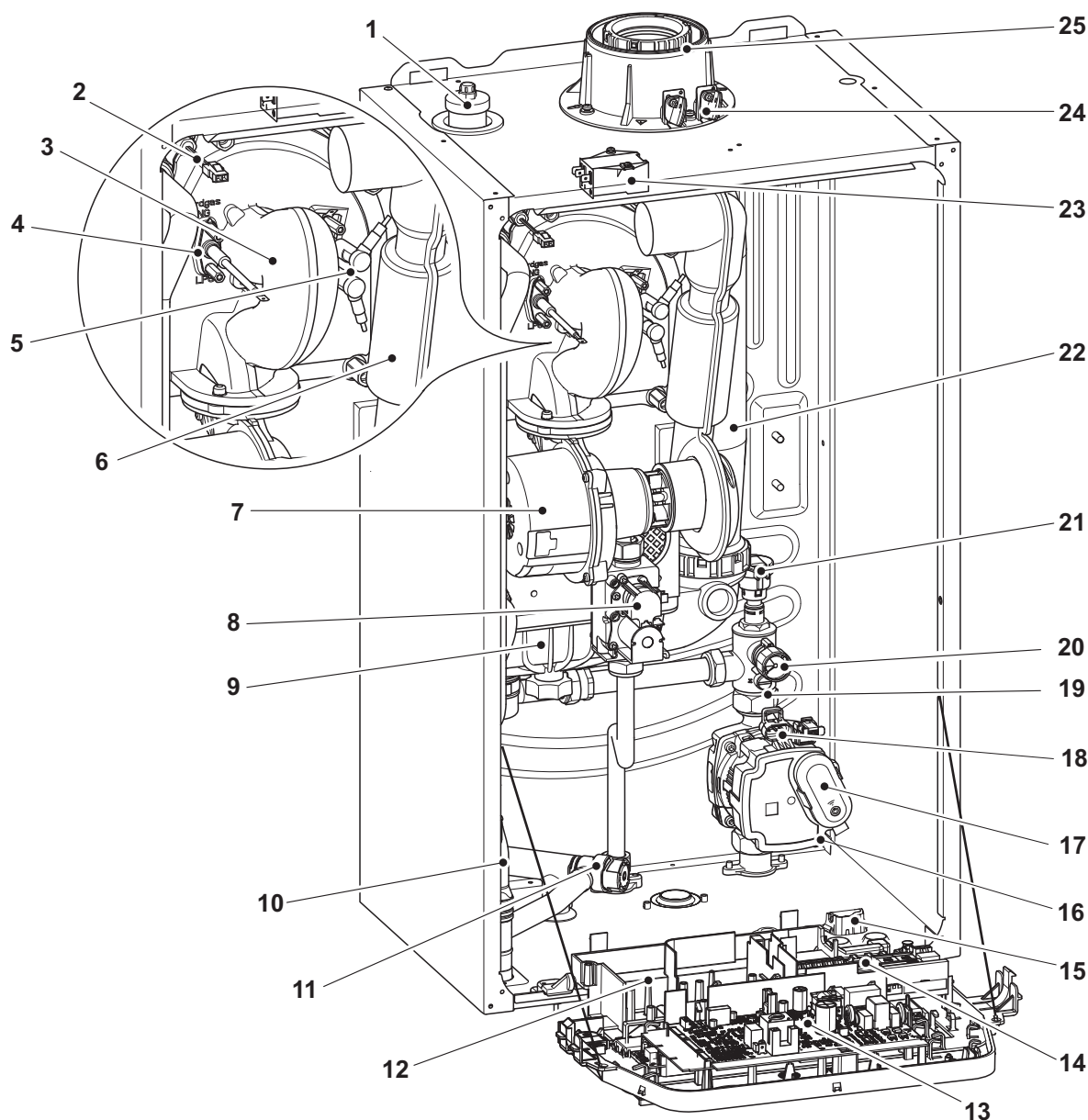
Rys.9 Widok kotła WGB (na rysunku bez przedniej obudowy i okrywy regulatora kotła)
