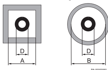
Rys.27 Minimalne wymiary przewodu kominowego
