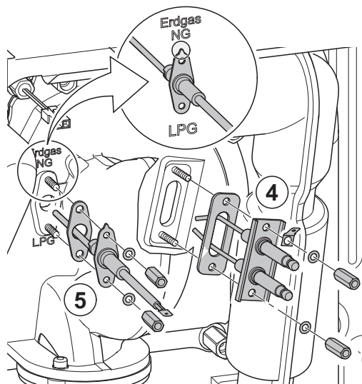
Rys.73 Wymontowywanie elektrody zapłonowej i jonizacyjnej
