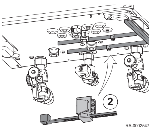
Rys.34 Montowanie opasek montażowych
