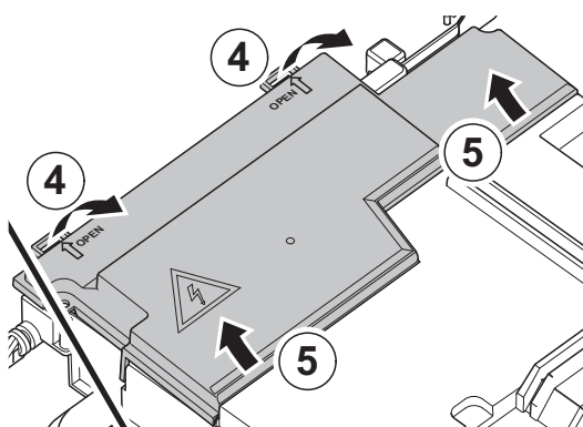
Rys.31 Zdejmowanie górnej osłony obudowy płytki obwodów drukowanych.
