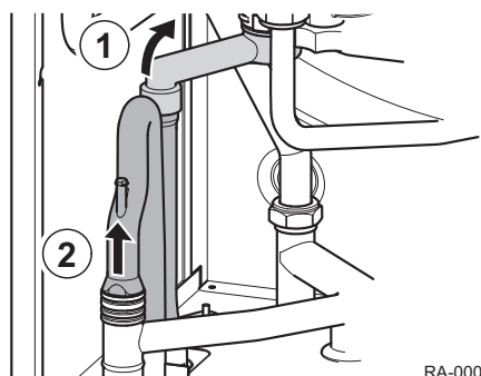
Rys.71 Wymontowywanie syfonu
