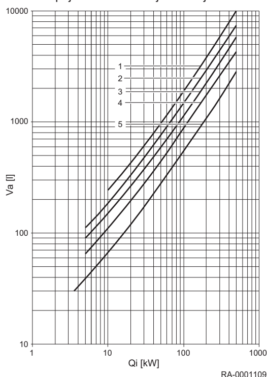
Rys.15 Określanie szacunkowej pojemności wodnej instalacji
