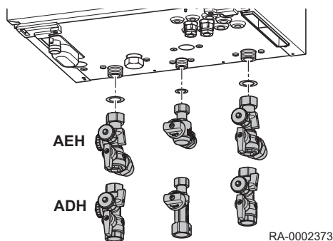
Rys.22 Montaż zaworów odcinających
