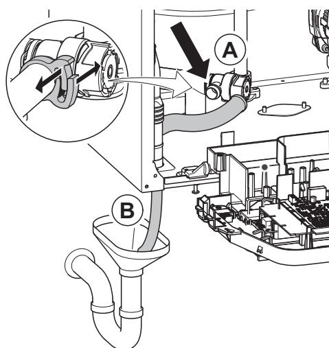
Rys.23 Zawór bezpieczeństwa i odprowadzenie kondensatu
