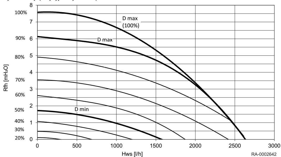
Rys.3 Dyspozycyjna wysokość podnoszenia WGB 38.2
