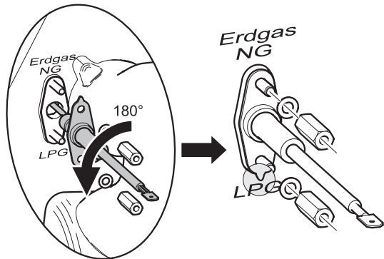
Rys.39 Zmiana rodzaju gazu na propan
