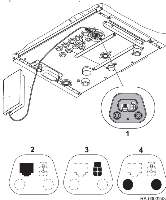
Rys.33 Położenie złącza
