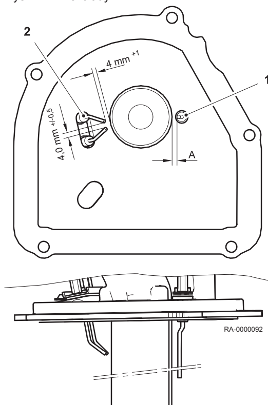
Rys.72 Elektrody
