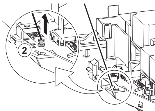
Rys.69 Odczepianie pasków przytrzymujących regulator
