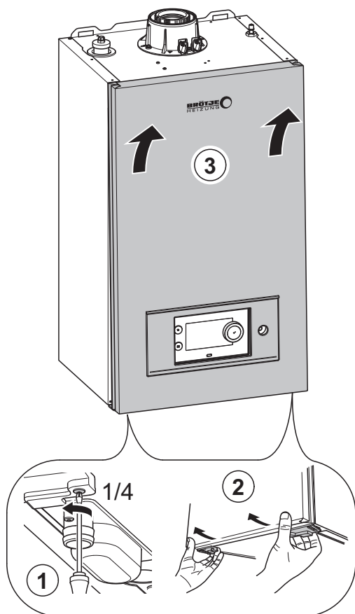
Rys.67 Zdejmowanie przedniej obudowy kotła
