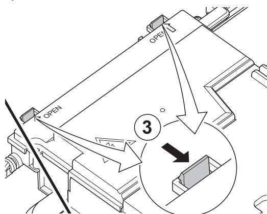
Rys.30 Otwieranie zatrzasków.
