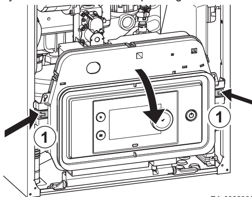
Rys.68 Zwalnianie zaczeów regulatora
