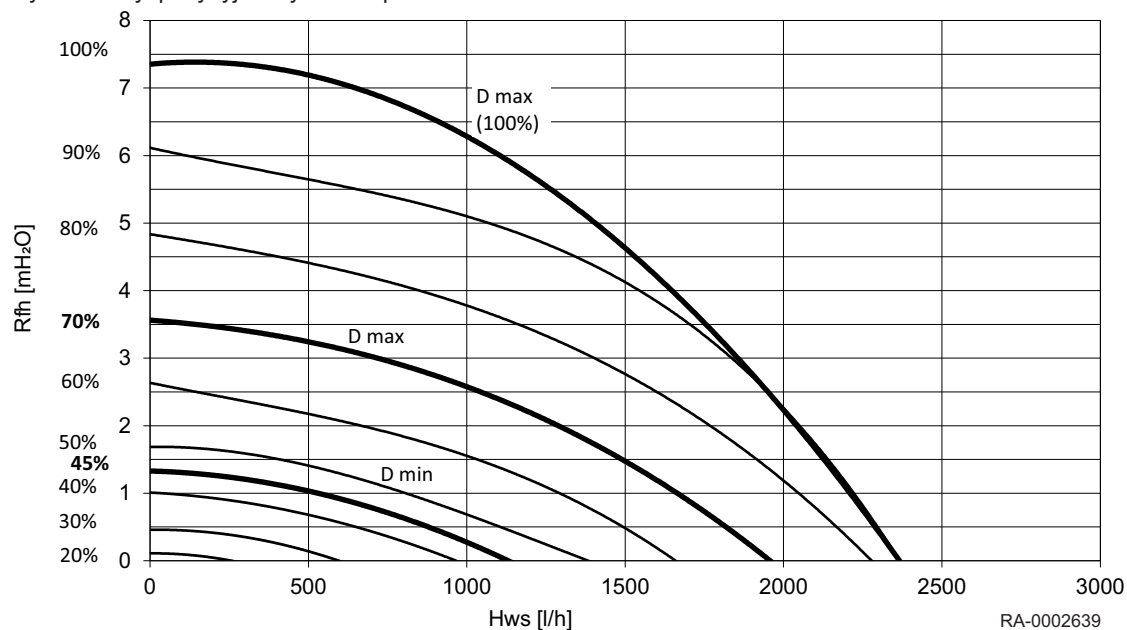
Rys.1 Dyspozycyjna wysokość podnoszenia WGB 14.2/WGB 22.2
