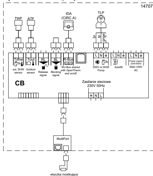
Rys.18 Schemat połączeń
