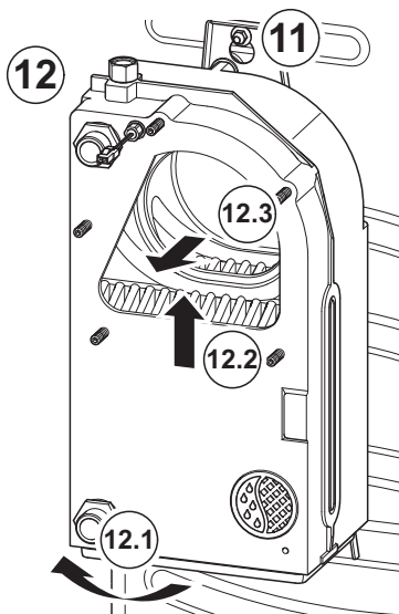
Rys.76 Wymontowywanie wymiennika ciepła
