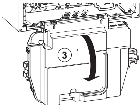
Rys.70 Wychylanie regulatora kotła całkowicie do dołu.
