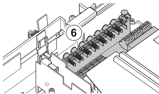
Rys.32 Płytki obwodów drukowanych, CB
