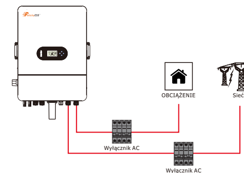
Rysunek 4.3-2 Podłączenie wyłącznika AC
