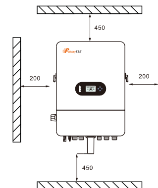
Rysunek 3.3-1 Przestrzeń instalacji falownika
