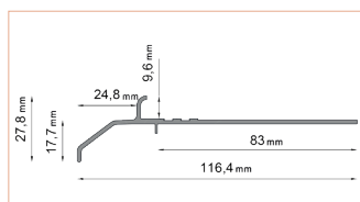
PROFIL OKAPOWY K20
