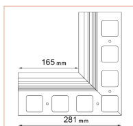
NAROŻNIK WEWNĘTRZNY K20 90
