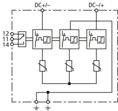
Schemat połączeń DCB YPV 1200 FM
