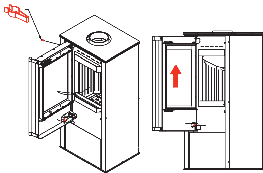
87. Schemat wymiany drzwi KOZA HATI / KOZA HATI door-replacement diagram / Schema für den Austausch der KOZA HATI-Tür / Схема замены дверцы KOZA HATI
