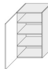
W4 50 (500/960/325)
