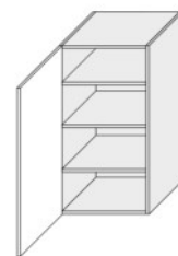
W4 45 (450/960/325)
