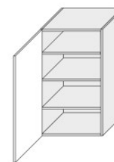
W4 60 (600/960/325)
