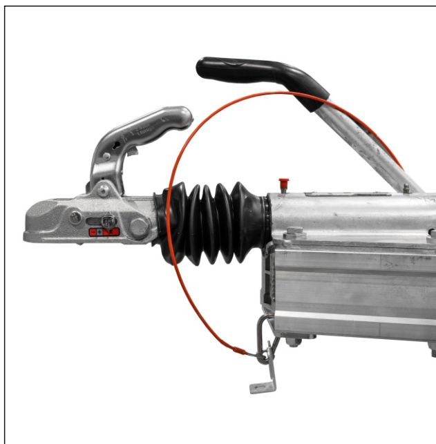
Urządzenie najazdowe z hamulcem postojowym
