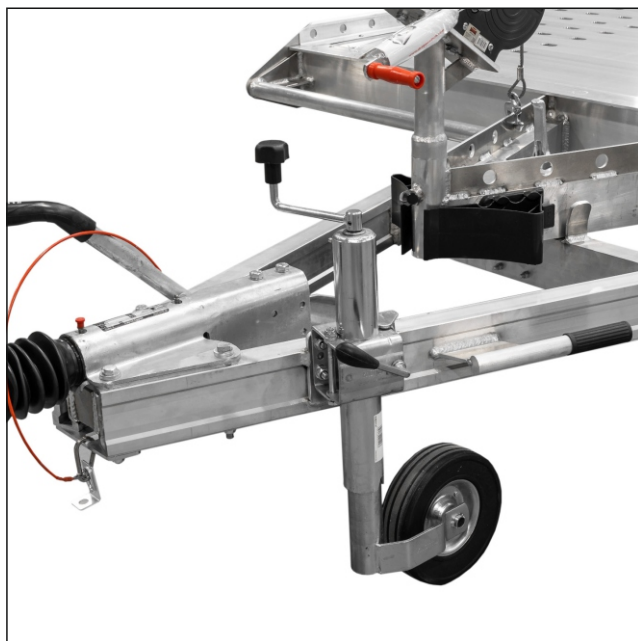
Solidne koło podporowe z gumową oponą i stalową felgą
