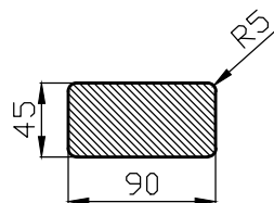
Przekrój A-A
