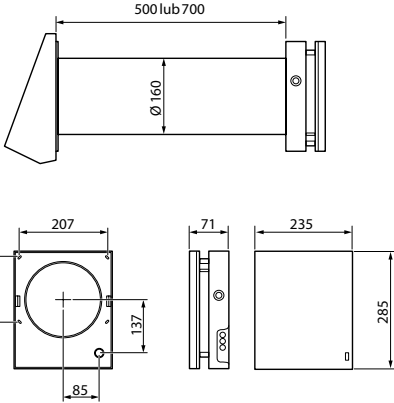
NIBE DVC 10
