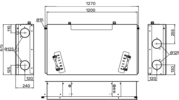
NIBE ERS 20-300
