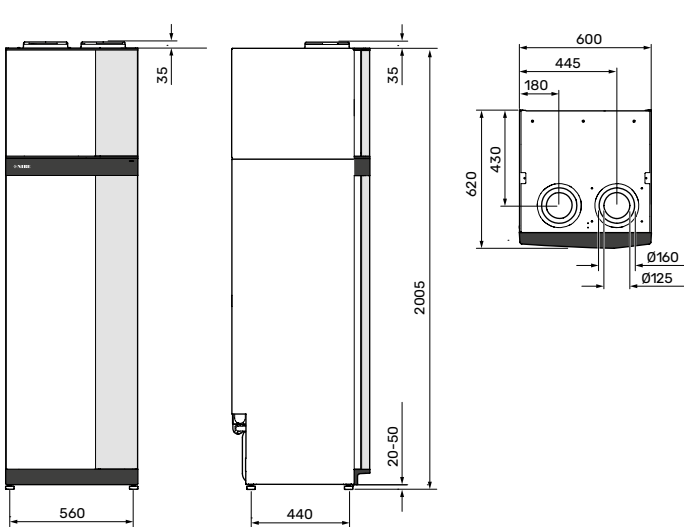
NIBE S735
