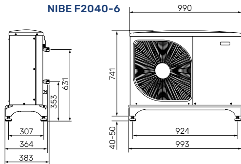
NIBE F2040-6
