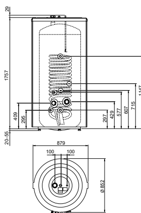
NIBE VPB 200
