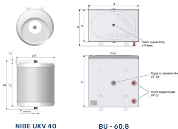
NIBE UKV 40
