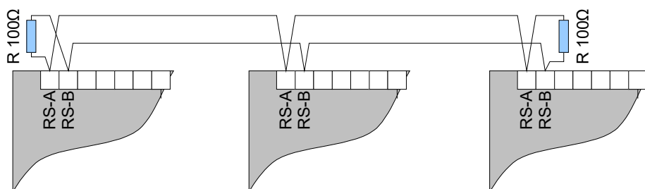
Rysunek 8: Przykładowy schemat prawidłowego połączenia interfejsu RS485
