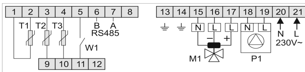
Rysunek 12: Rozmieszczenie wyprowadzeń BWC 310
