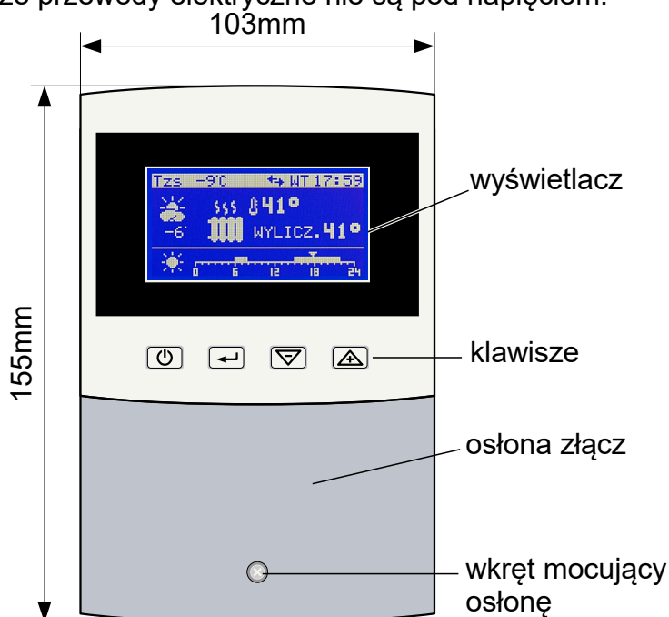
Rysunek 10: Budowa i wymiary termostatu BWC 310
