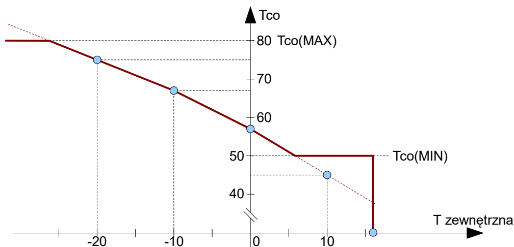
Rysunek 4: Przykładowa charakterystyka grzewcza
