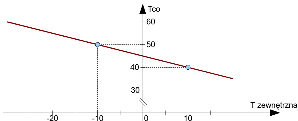
Rysunek 5: Przykładowa charakterystyka temperatury zadanej powrotu w funkcji temperatury zewnętrznej
