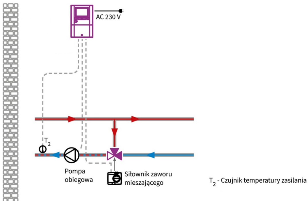
Rysunek 2: Regulacja temperatury za pomocą zaworu trójdrogowego na powrocie do źródła ciepła
