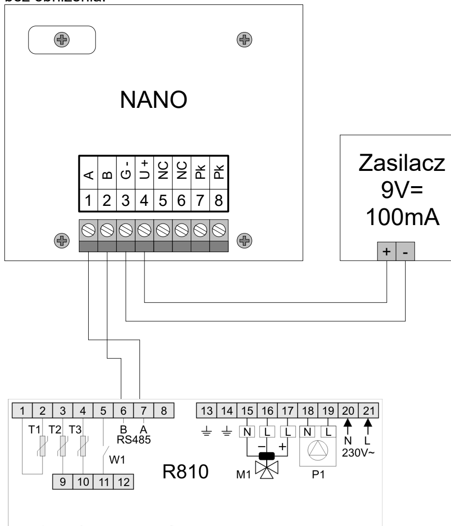
Rysunek 9: Schemat podłączenia BWC 310 do termostatu pokojowego NANO
