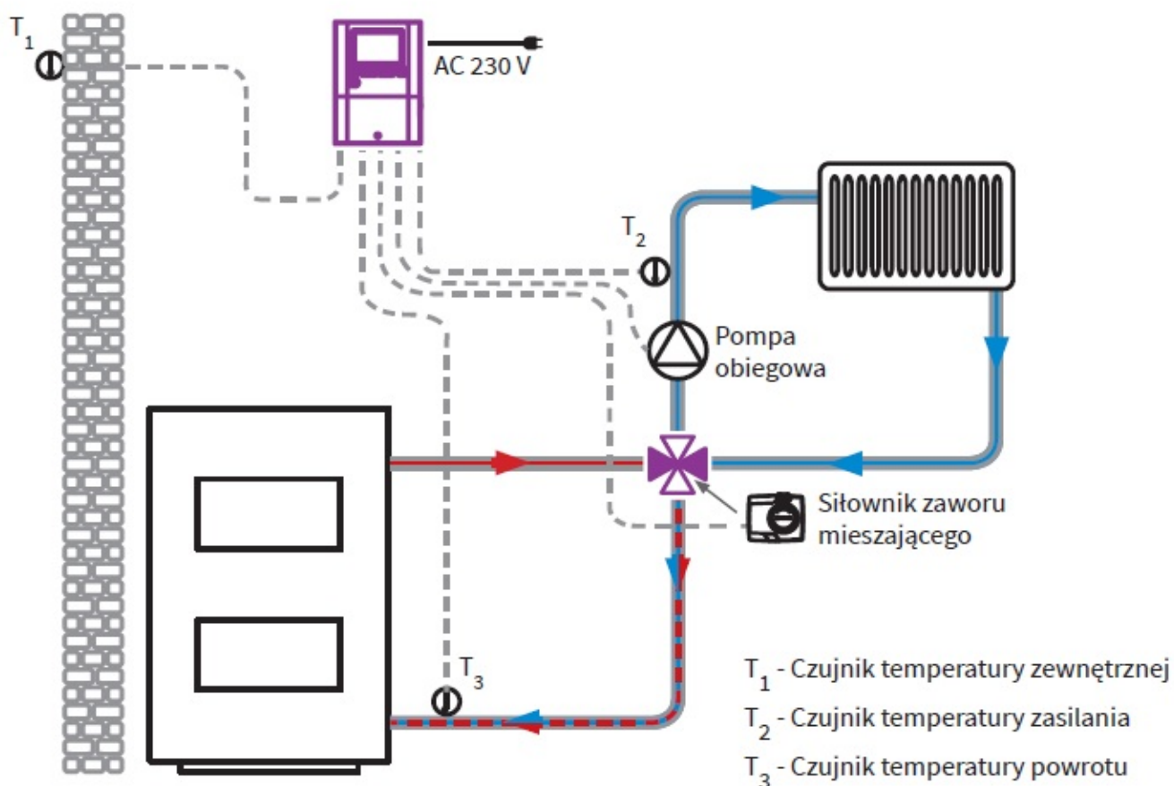
Rysunek 7: Schemat instalacji z zaworem 4-drogowy
