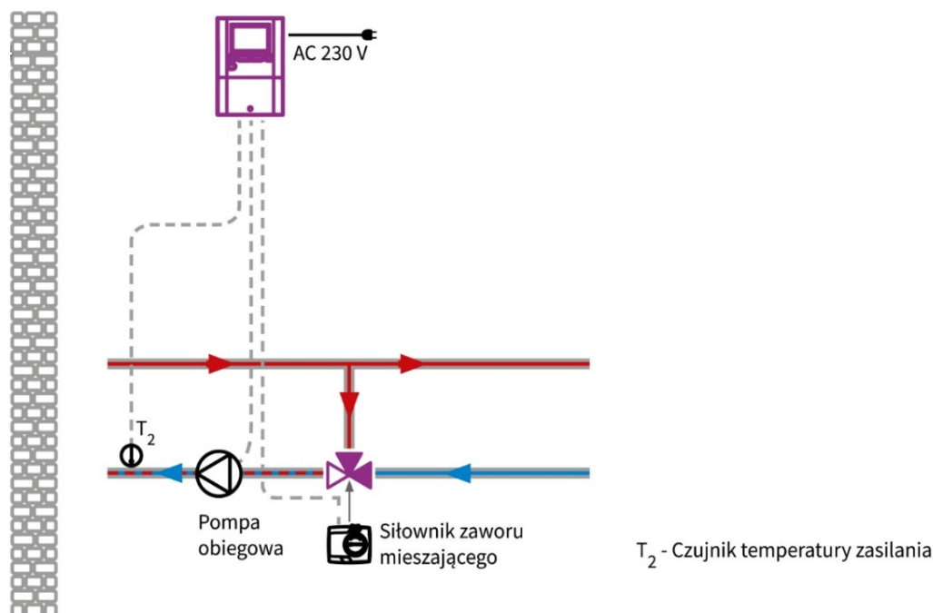
Rysunek 6: Ochrona kotła przed niską temperaturą powracającą do kotła
