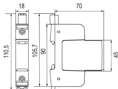
ETITEC ML T123 300/12,5 1+0, 1+1
