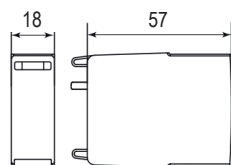
Moduł wymienny ETITEC ML T123 300/12,5
