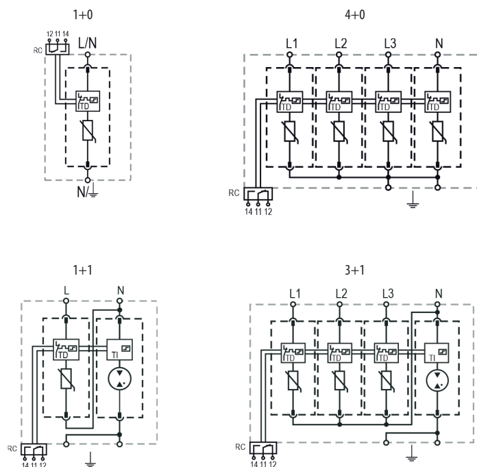
Układy wewnętrzne ETITEC ML T123 300/12,5 RC
