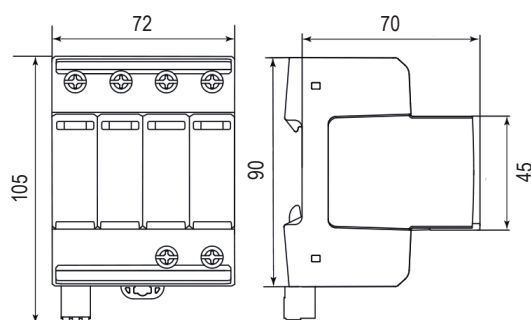
ETITEC ML T123 300/12,5 4+0, 3+1
