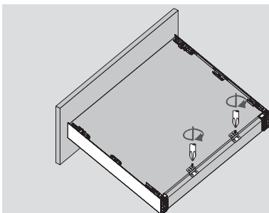
Montaż wsporników mocujących Fixing-brackets assembly
