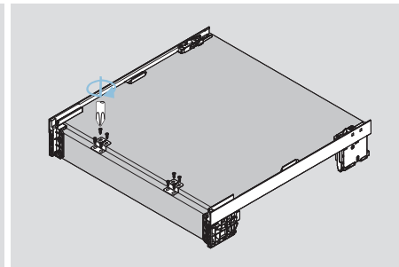
Montaż wsporników mocujących Fix-brackets assembly
