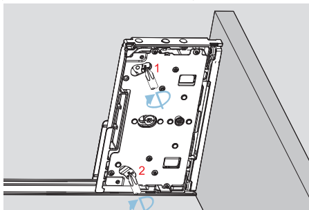
Użyj śrubokręta by zwolnić blokadę 1, a następnie zwolnij blokadę 2, zdejmij front szuflady Turn screw driver to release lock 1, then release lock 2, remove the drawer front
