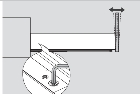
Regulacja nachylenia (kluczem imbusowym M3) Tilt adjustmant (by M3 Allen key)
