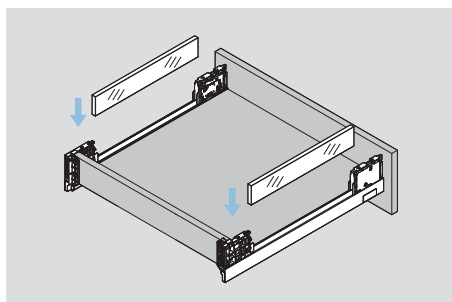
Wstaw szklane boki Insert glass-boxside
