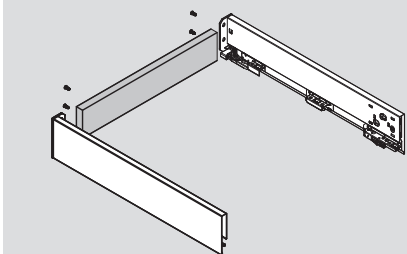
Montaż tylnej ścianki Back assembly
