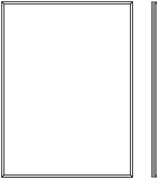
WZÓR 1 SPECYFIKACJA: ramka 10mm, zagłębienie 5mm WYKOŃCZENIE: fornir
