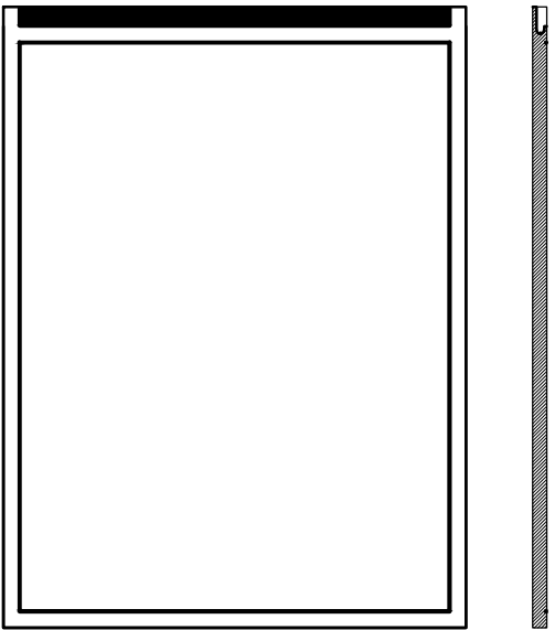
WZÓR 6 SPECYFIKACJA: MDF barwiony w masie (kolor czarny) uchwyt "J" frezowany ramka frezowana WYKOŃCZENIE: fornir
