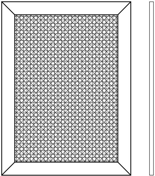
WZÓR 3 SPECYFIKACJA: ramka 60mm WYKOŃCZENIE: fornir, plecionka wiedeńska
