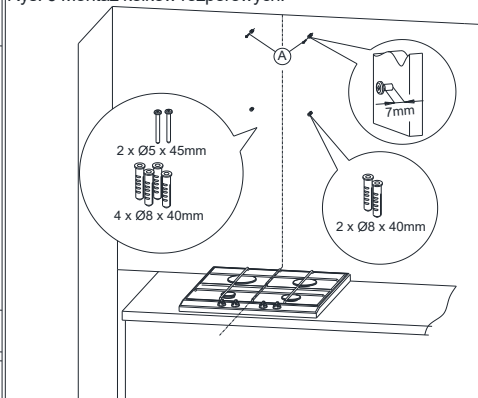
Rys. 8 Zawieszanie uchwytu mocowania okapu.
