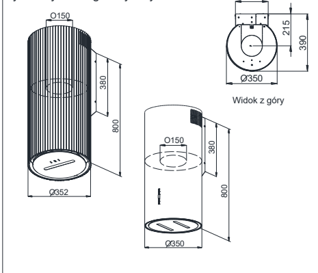
Rys. 2 Rysunek gabarytowy.
