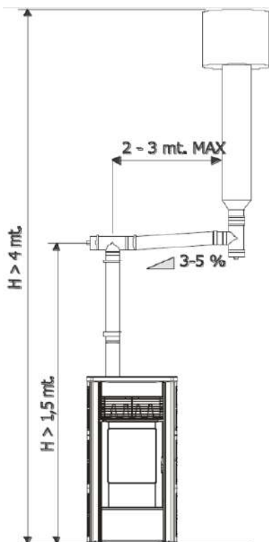
Installationsbeispiel eines Pelletofens
