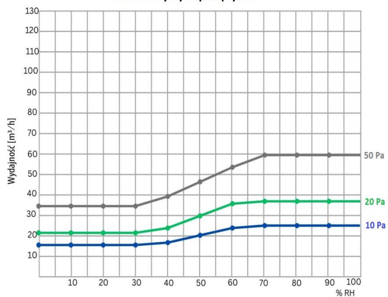
Charakterystyka przepływu
