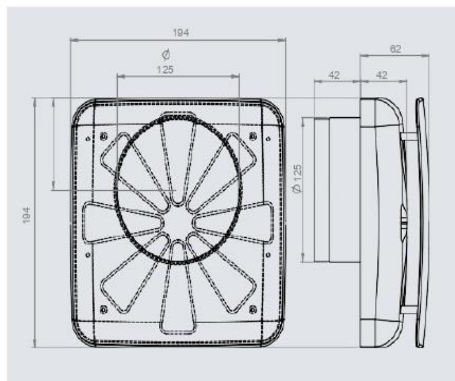
Wymiary kratki wentylacyjnej (mm).
