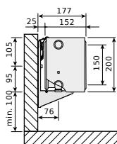
Plint, typ 33 z zawieszzeniami ściennymi Monclac, widok z boku
