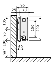
Plint, typ 21s z zawieszaniami ściennymi Monclac, widok z boku
