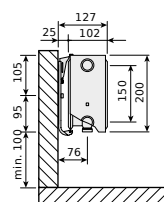
Plint, typ 22 z zawieszaniami ściennymi Monclac, widok z boku
