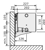
Plint, typ 44 z zawieszzeniami ściennymi Monclac, widok z boku
