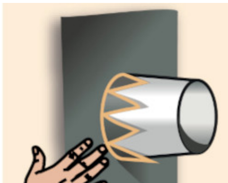
Rysunek 2 – Następnie umieścić pierwszy wycięty kawałek membrany wokół elementu
