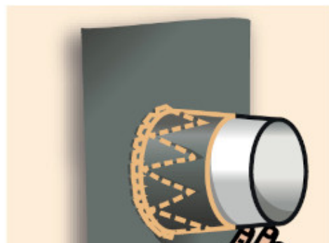
Rysunek 3 – Umieszczenie drugiego kawałka Mapethene LT tak, aby powstał kołnierz izolacyjny wokół elementu przechodzącego
