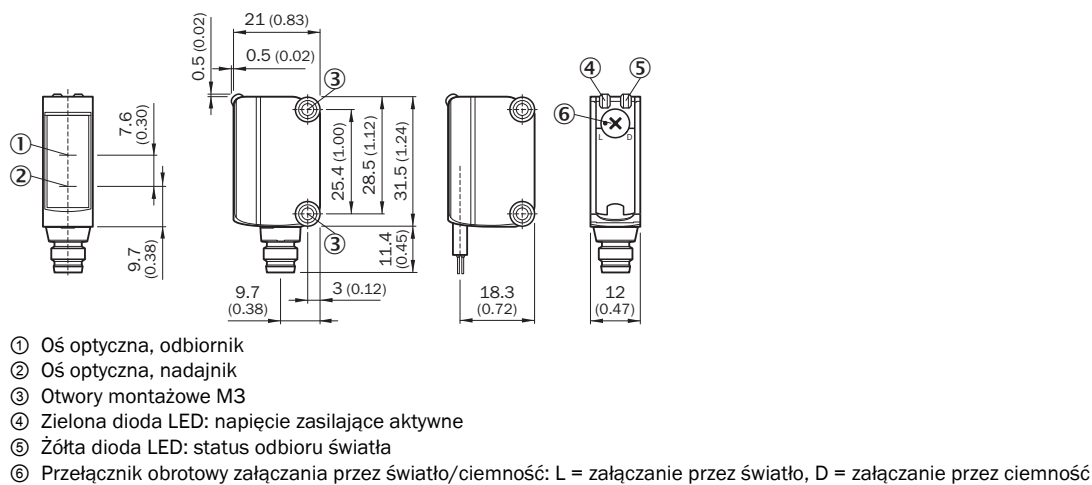
Rysunek wymiarowy (Wymiary w mm)
