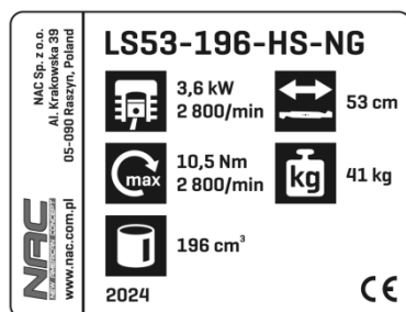
Tabliczka znamionowa
