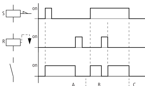
Rys. 92: Wykres działania "Ustawiania" i "Kasowania"
