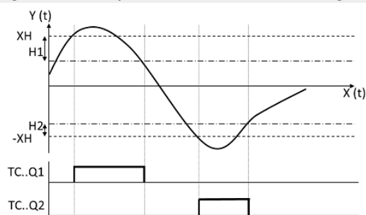
Rys. 198: Wykres działania regulatora trójpunktowego
