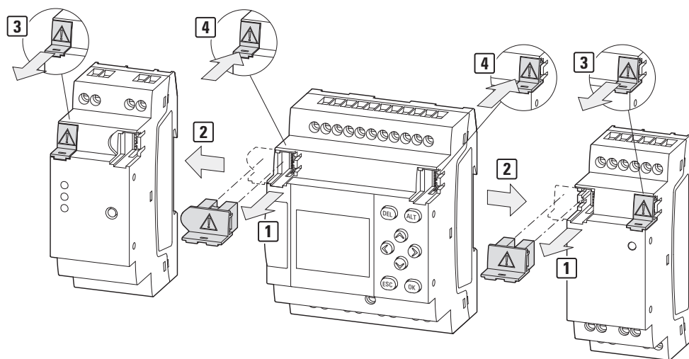
Rys. 10: Usunąć sąsiednie wtyczki połączeniowe
