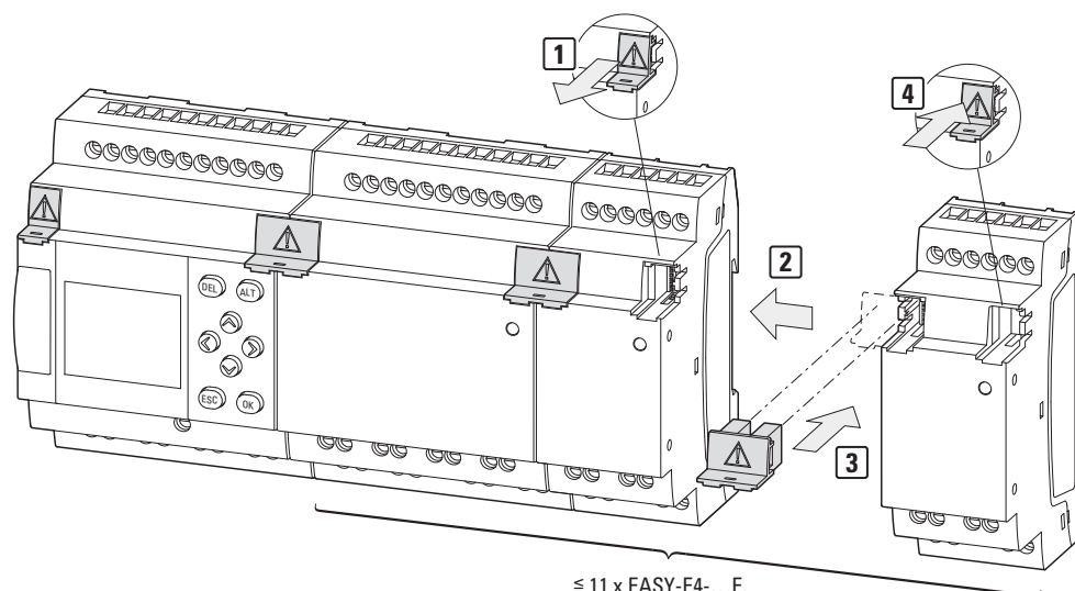
Rys. 5: Montaż urządzenia podstawowego z rozszerzeniami.
