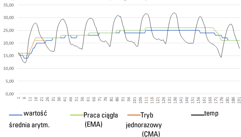
Rys. 175: Przykładowa godzinowa krzywa charakterystyki pomiarów temperatury w okresie 7 dni
