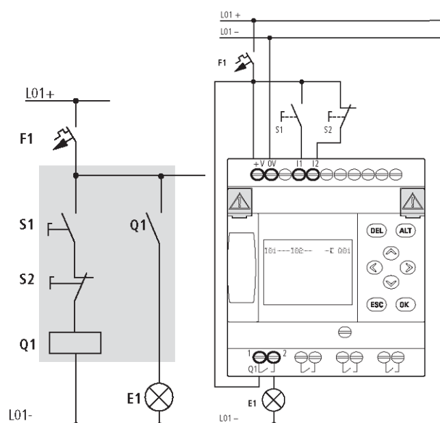
Rys. 76: Wysterowanie lamp
