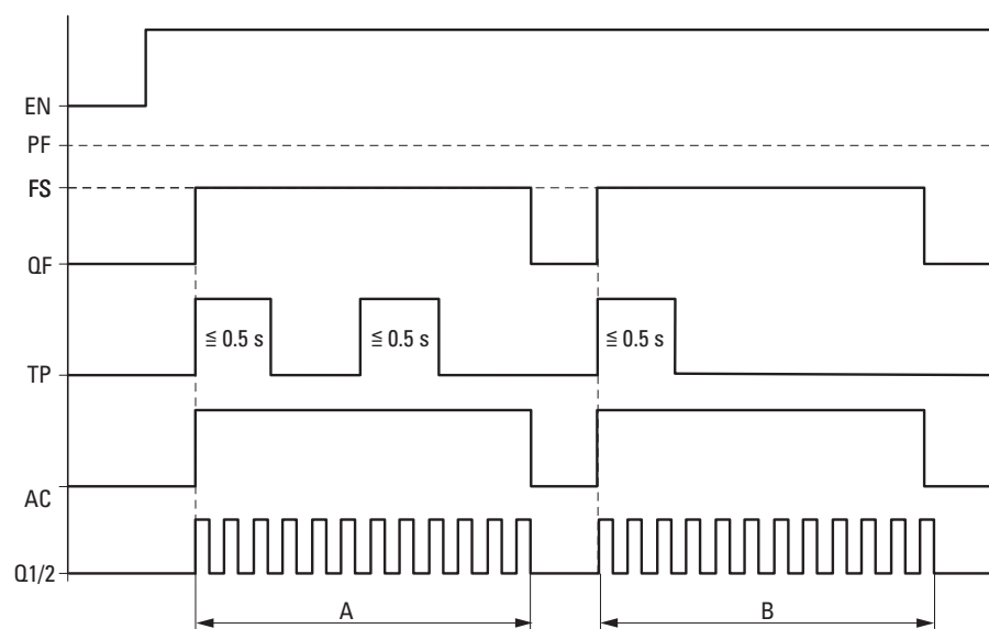
Rys. 193: Wykres działania impulsowania z zadaną liczbą kroków P1
