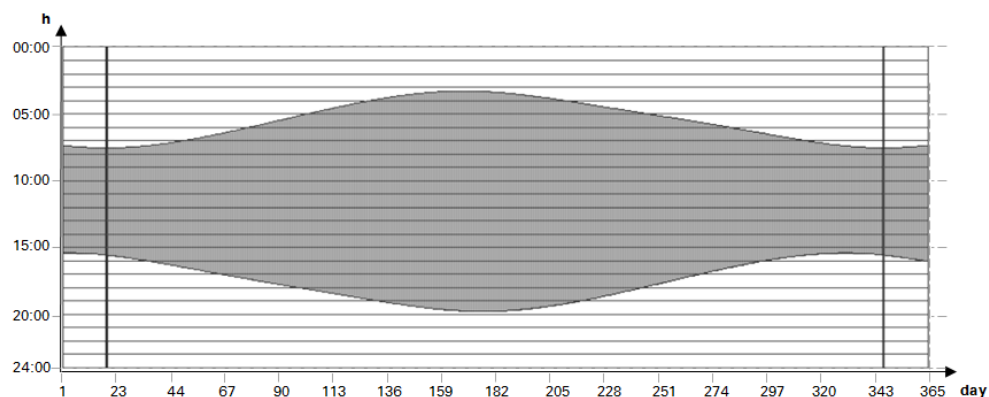
Rys. 159: Brak offsetu; O1=0; O2=0; Q1=1 między wschodem a zachodem słońca
