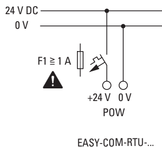
Rys. 341: Podłączyć zasilanie EASY-COM-RTU-...
