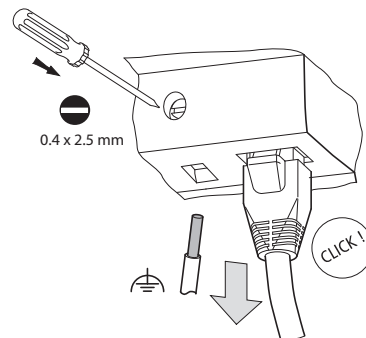
Rys. 34: Usuwanie kabla Ethernet
