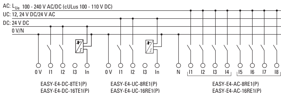
Rys. 15: Podłączanie wejść cyfrowych rozszerzeń
