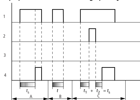
Rys. 138: Wykres działania przekaźnika czasowego o opóźnionym zadziałaniu (z losowym przełączaniem/bez)
