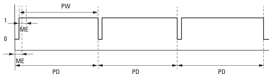
Rys. 184: Na wyjściu modułu wyświetlany jest sygnał ciągły przy SV = 3768, ME = 93 ms, PD=1000 ms; E1 = 1
