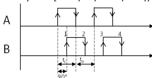
Rys. 168: Moduł funkcyjny CI zliczający do przodu; QV=QV+4
