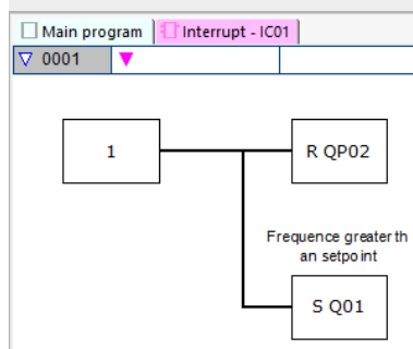
Rys. 257: Program przerwania easySoft 8 Pomiar częstotliwości
