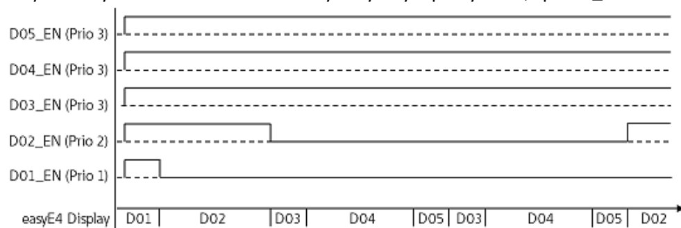
Rys. 220: Wykres działania znaczników tekstowych z modułami tekstowymi o tym samym priorytecie, 3
