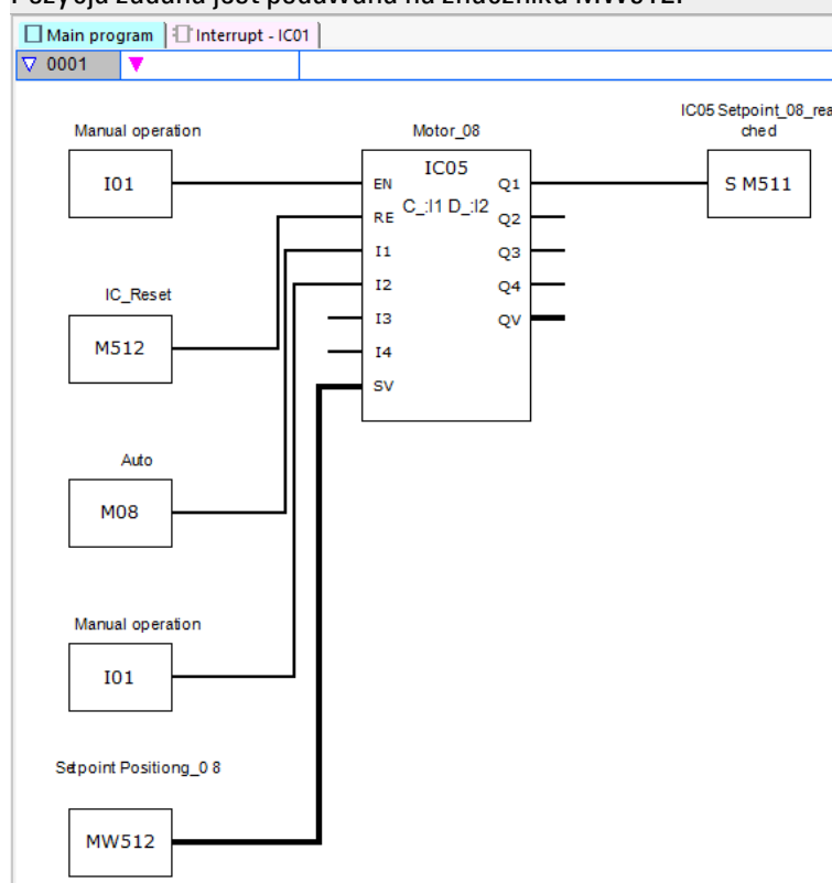
Rys. 254: Program główny easySoft 8 Moduł licznika przyrostowego
