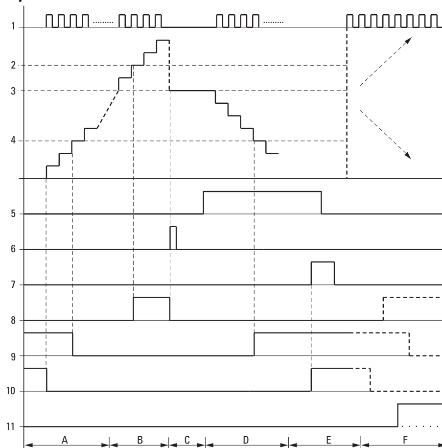
Rys. 165: Wykres działania modułu licznika
