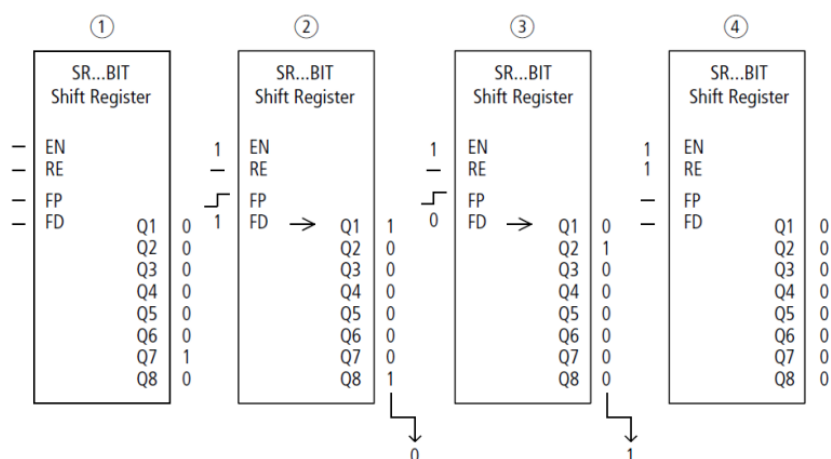
Rys. 212: Rejestr przesuwany SR...: operacja do przodu w trybie pracy BIT
