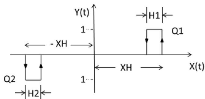
Rys. 197: Wykres czasowy regulatora trójpunktowego
