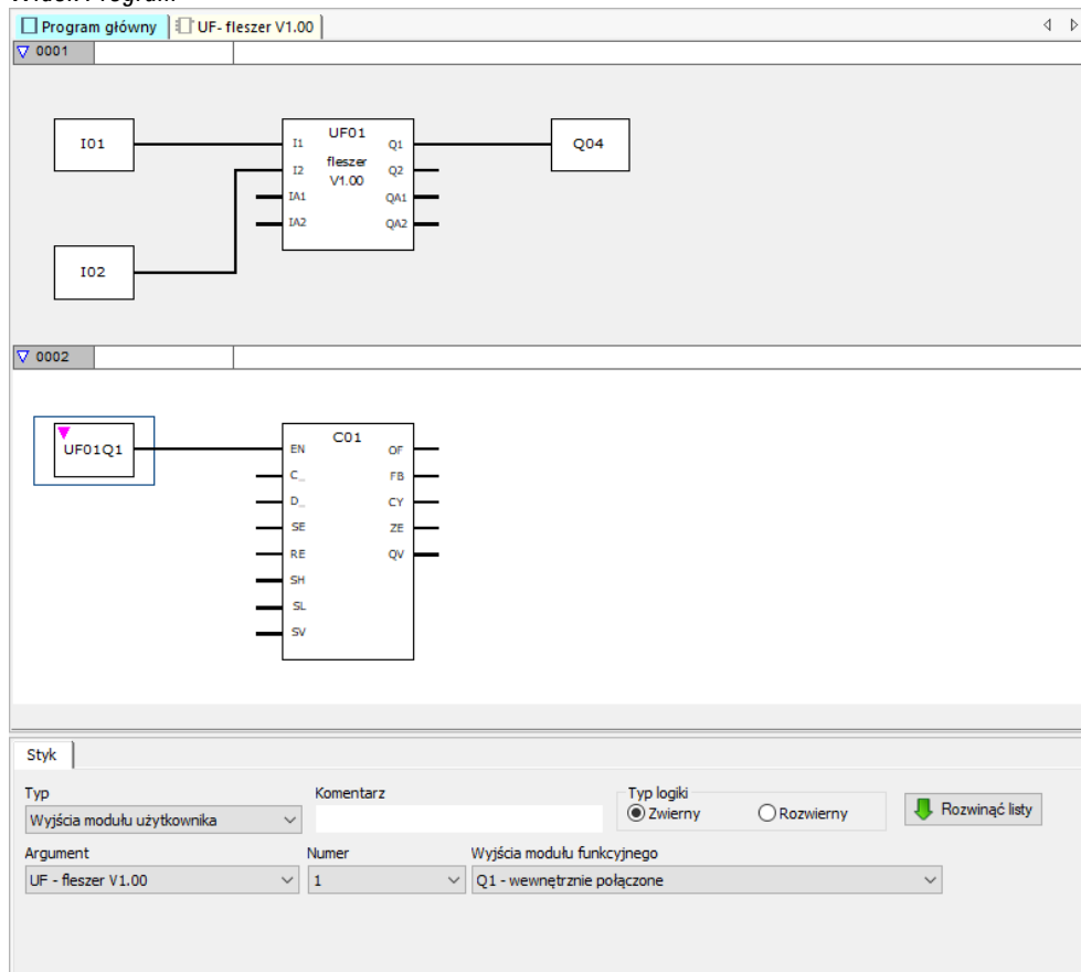
Rys. 271: Oprzewodowanie wejść/wyjść
