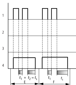
Rys. 141: Wykres działania przekaźnika czasowego z opóźnionym opadaniem (z losowym przełączaniem/bez, z ponownym wyzwaniem/bez)
