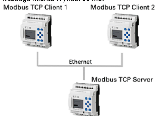
Rys. 343: Jedno urządzenie easyE4 jako serwer Modbus TCP obsługuje dwa klienty Modbus TCP
