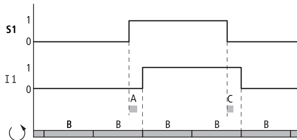
Rys. 300: Procedura łączenia przy dezaktywowanej zwłoce na wejściach I
