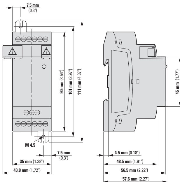
Rys. 361: Wymiary w mm (calach)
