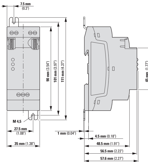
Rys. 363: Wymiary w mm (calach) - rozszerzenia 2TE
