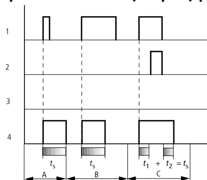
Rys. 143: Wykres działania przełącznika czasowego, formowanie impulsu 1
