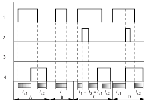
Rys. 142: Wykres działania przełącznika czasowego, z opóźnionym zadziałaniem i opadaniem
