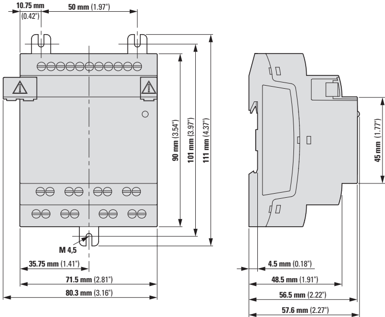
Rys. 359: Wymiary w mm (calach) - rozszerzenia 4TE
