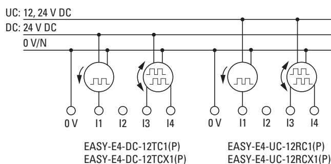
Rys. 16: Podłączanie cyfrowych wejść zliczających
