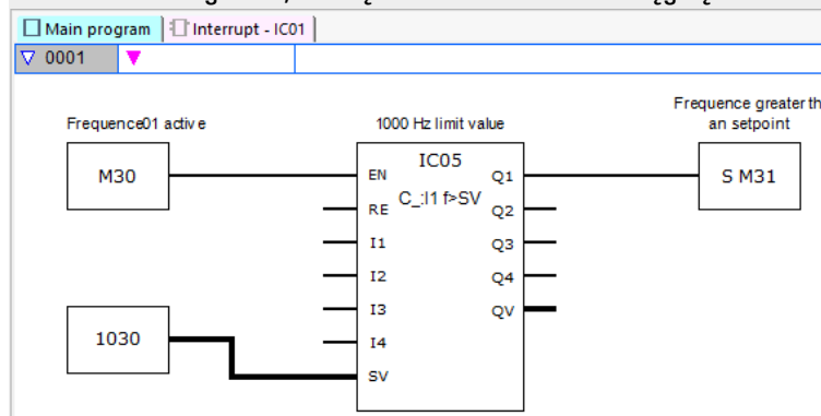
Rys. 256: Program główny easySoft 8 Pomiar częstotliwości
