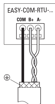
Rys. 340: EASY-COM-RTU-... Podłączanie wyjść
