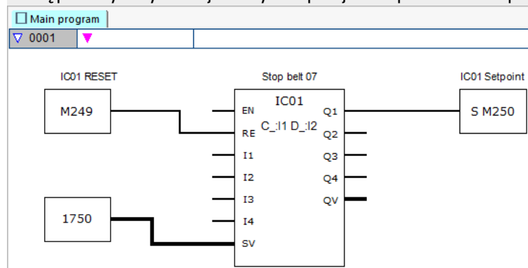
Rys. 250: Program główny easySoft 8 Licznik impulsów z zewnętrznym sterowaniem kierunkiem
