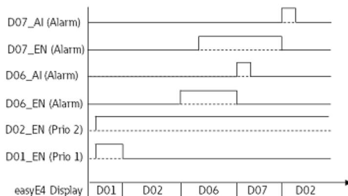
Rys. 219: Wykres działania wyświetlania tekstu
