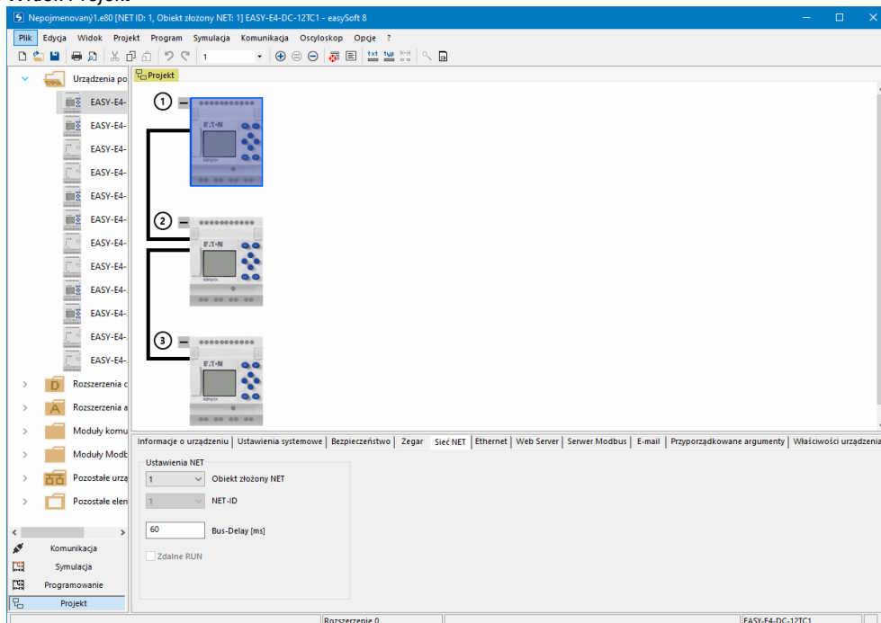
Rys. 307: Konfiguracja sieci NET z projektem i programem
