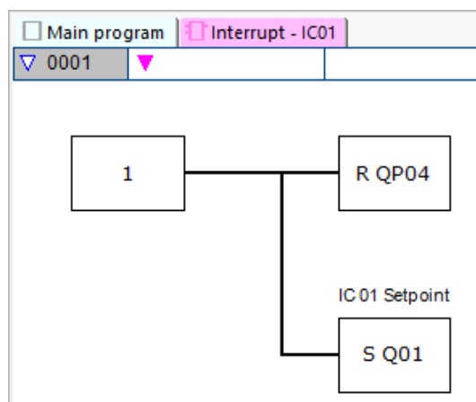
Rys. 251: Program przerwania easySoft 8 Licznik impulsów z zewnętrznym sterowaniem kierunkiem
