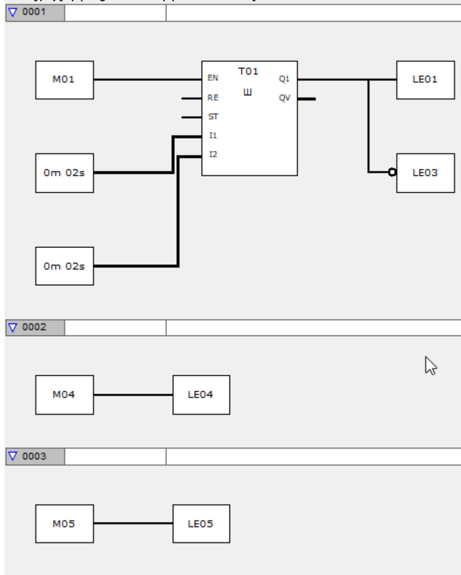
Rys. 296: Widok programu/przykładowy program w FBD
