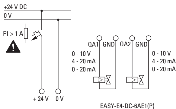
Rys. 24: Podłączanie wyjść analogowych EASY-E4-DC-6AE1(P)
