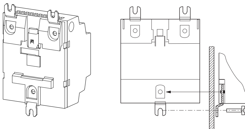
Rys. 9: Przykład: montaż urządzenia 4TE za pomocą śrub
