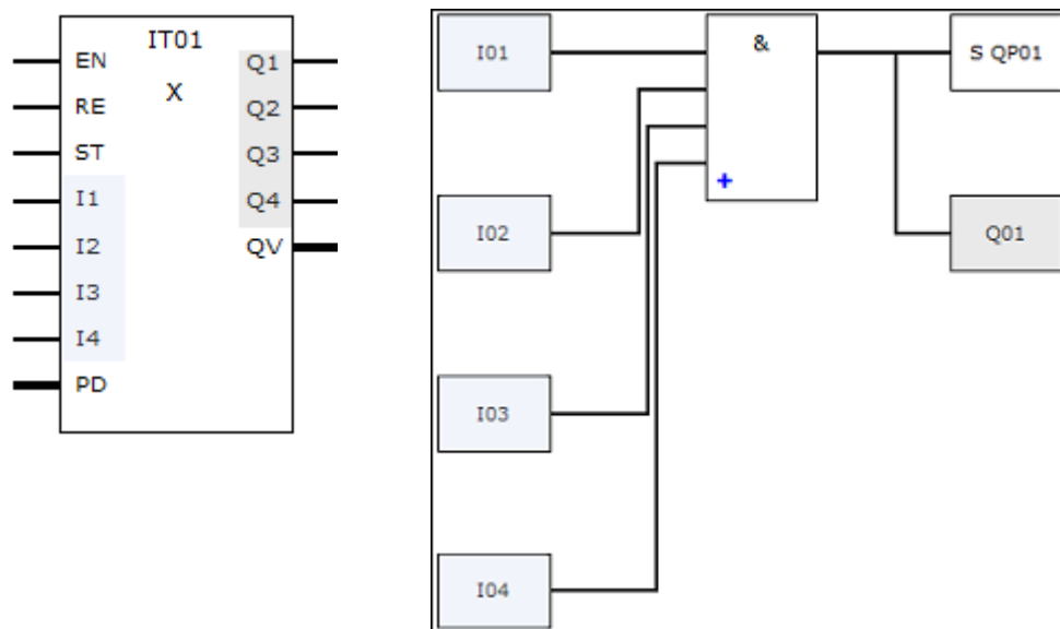
Rys. 261: Przekazywanie stanów wejść i wyjść między programem głównym a programem przerwania
