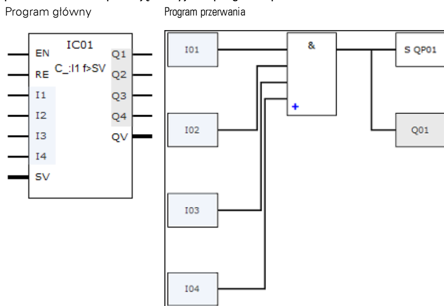
Rys. 249: Przekazywanie stanów wejść i wyjść między programem głównym a programem przerwania
