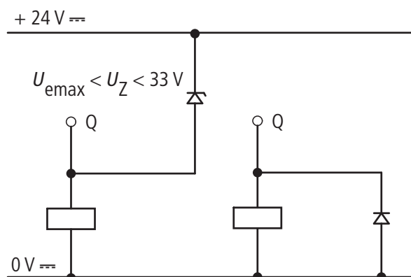
Rys. 21: Obciążenie indukcyjne z połączeniem ochronnym
