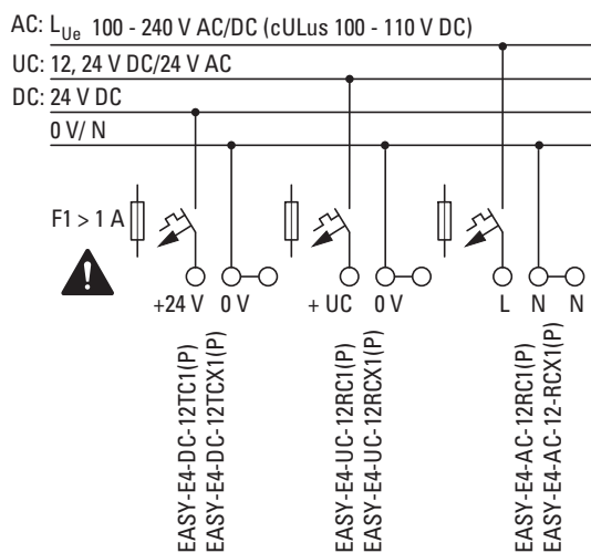
Rys. 12: Podłączanie zasilania urządzeń podstawowych
