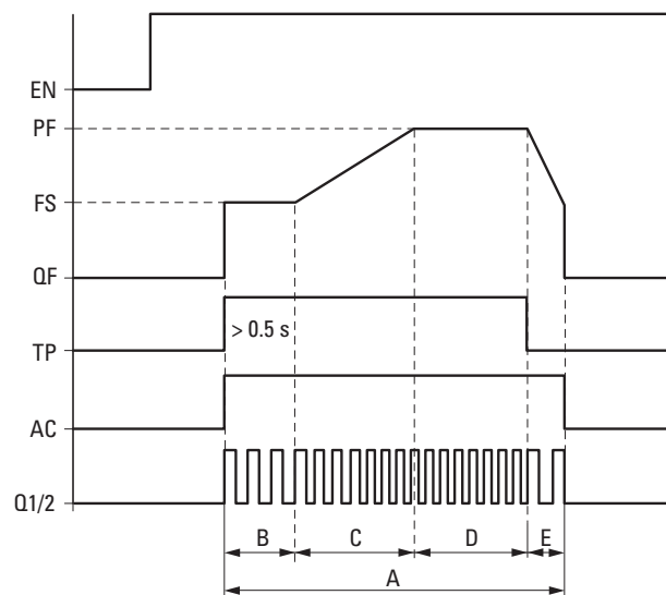
Rys. 194: Wykres działania impulsowania z zadana częstotliwością impulsowania, P1 osiągnięte po fazie hamowania
