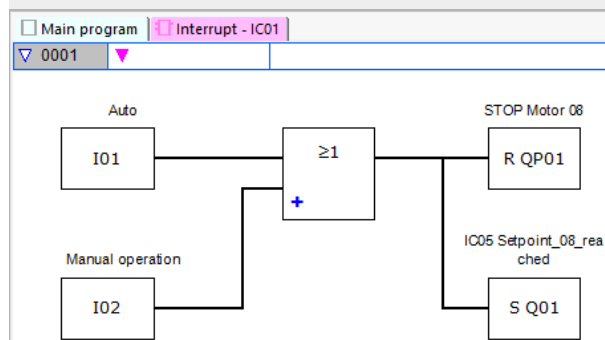
Rys. 255: Program przerwania easySoft 8 Moduł licznika przyrostowego
