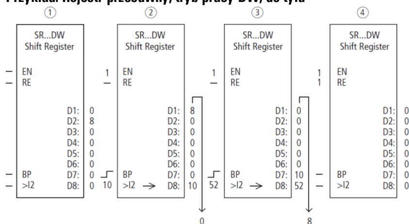
Rys. 213: Rejestr przesuwany SR...: operacja do tyłu w trybie pracy DW
