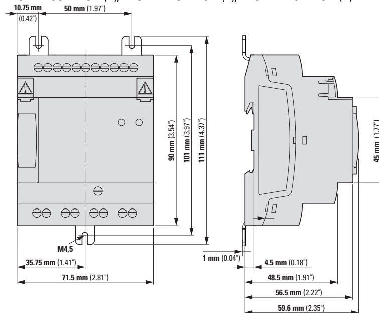
Rys. 358: Wymiary w mm (calach) Urządzenia podstawowe EASY-E4-...-12...CX1(P)
