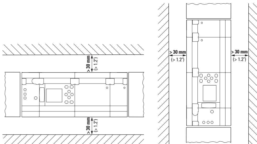
Rys. 4: Odstęp minimalny 3 cm
