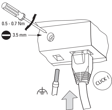
Rys. 32: Podłączanie kabla Ethernet
