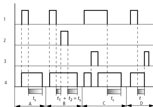
Rys. 140: Wykres działania przekaźnika czasowego z opóźnionym opadaniem (z losowym przełączaniem/bez, z ponownym wyzwaniem/bez)
