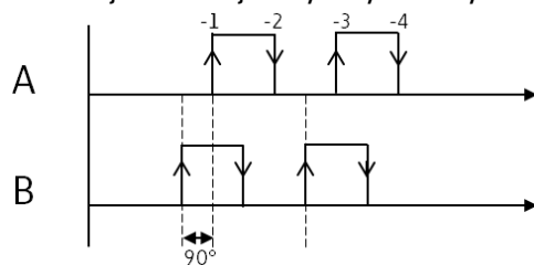
Rys. 169: Moduł funkcyjny CI zliczający do tyłu; QV=QV-4
