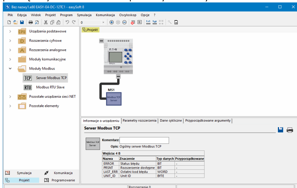
Rys. 345: Pulpit roboczy z urządzeniem podstawowym i modułami serwera Modbus TCP.
