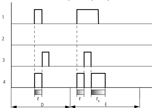
Rys. 144: Wykres działania przełącznika czasowego, formowanie impulsu 2
