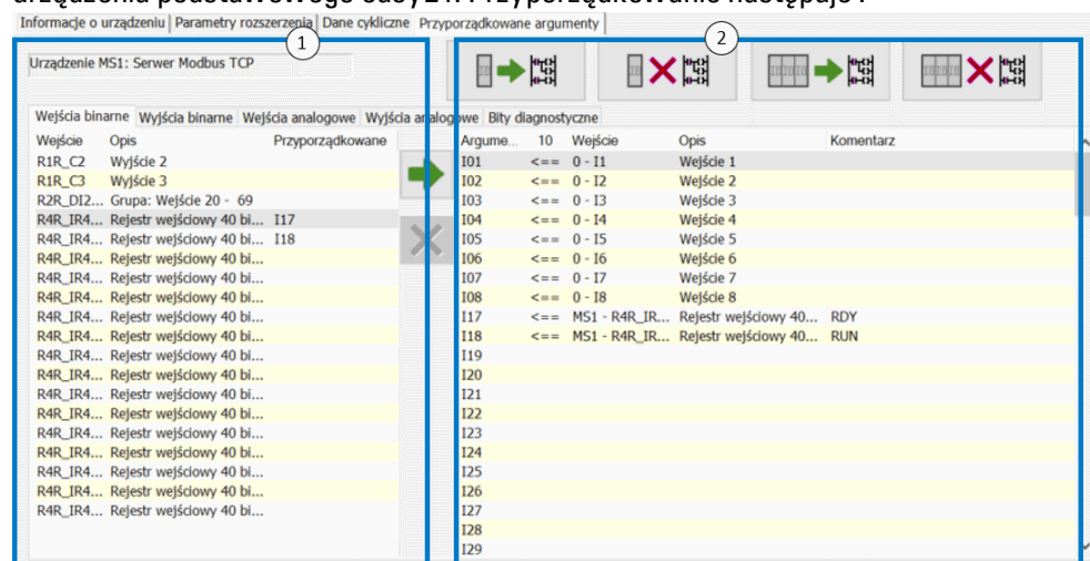
Rys. 351: Zakładki Przyporządkowane argumenty wg definicji FC1, FC2 i FC4; wejścia bitów R4R_IR40x0 i R4R_IR40x1 zostały już przyporządkowane do argumentów urządzenia podstawowego I17 i I18.
