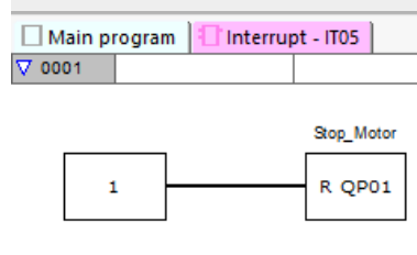
Rys. 263: Program przerwania easySoft 8 - sterowany czasowo
