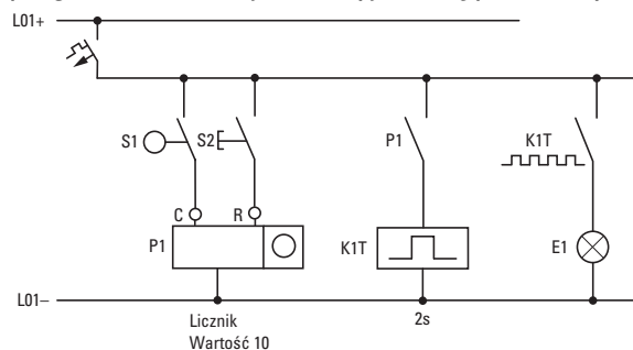
Rys. 282: Stałe oprzewodowanie z przekaźnikiem
