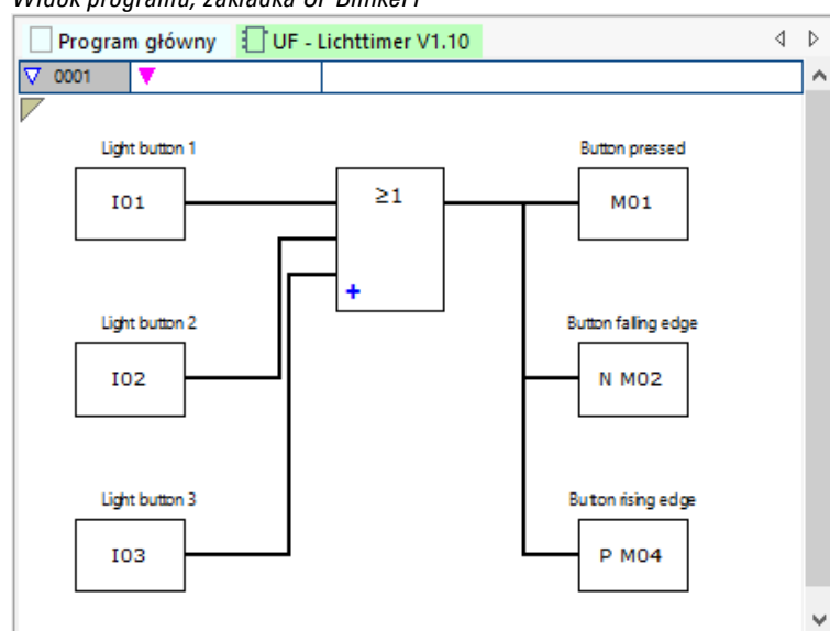
Rys. 268: Widok programu, moduł użytkownika UF Blinker1
