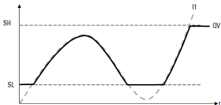
Rys. 199: Rysunek: Obcinanie wartości wejściowej na poziomie ustalonej granicy
