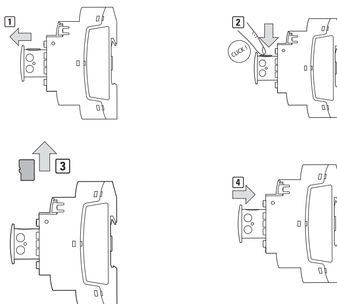
Rys. 30: Usuwanie karty pamięci
