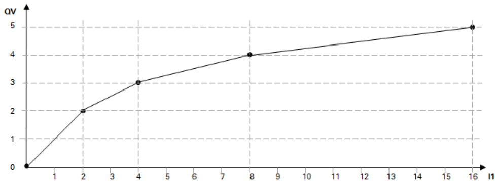
Rys. 181: Przykład krzywej charakterystyki dla modułu funkcyjnego PM
