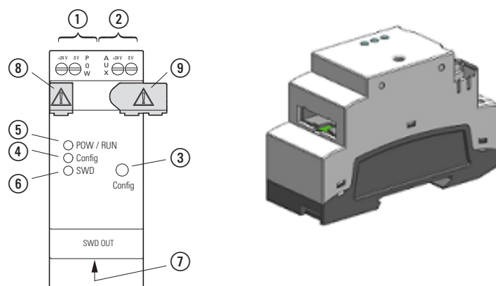
Rys. 334: Wersja urządzenia w 2TE
