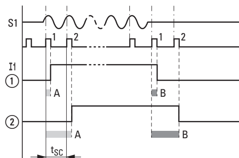
Rys. 301: Czasy opóźnienia przy analizie sygnału wejściowego AC
