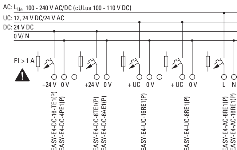
Rys. 13: Podłączanie zasilania rozszerzeń
