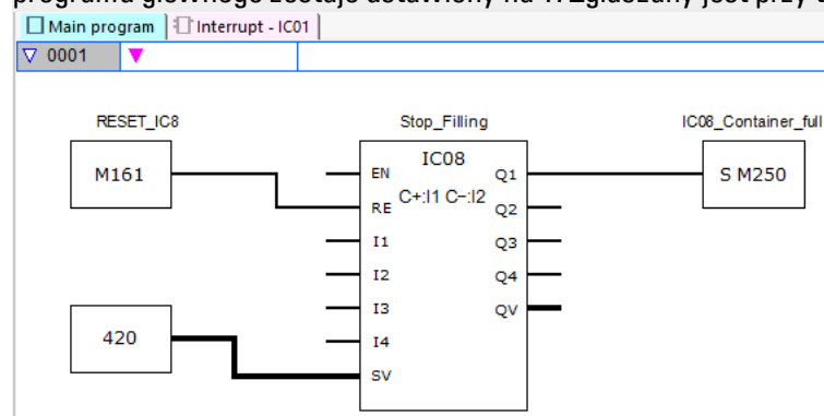
Rys. 252: Program główny easySoft 8 - dwa wejścia zliczające
