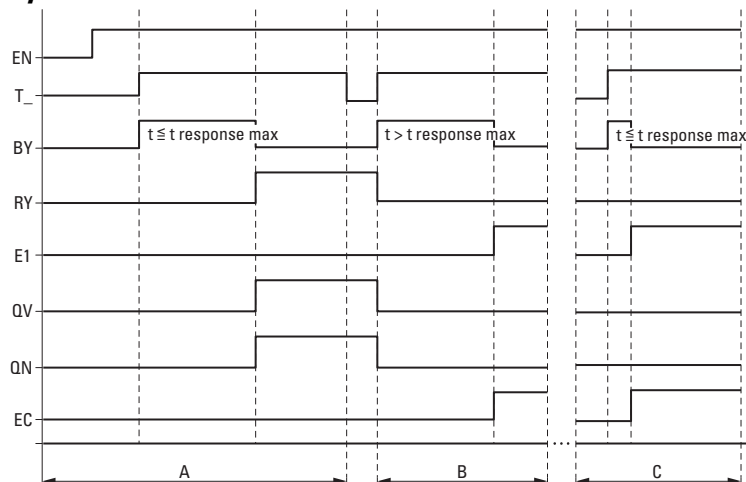
Rys. 244: Wykres działania licznika częstotliwości
