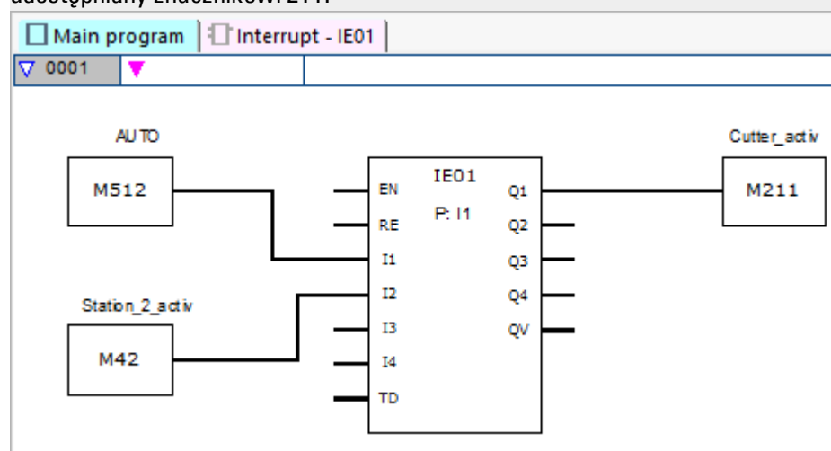
Rys. 259: Program główny easySoft 8- sterowania na podstawie zbocza
