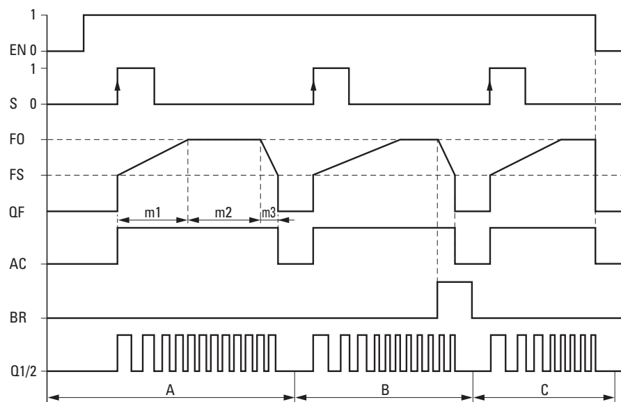
Rys. 192: Wykres działania wyjścia impulsowego PO przy zadanej liczbie impulsów I1 – możliwe fazy w normalnym trybie pracy
