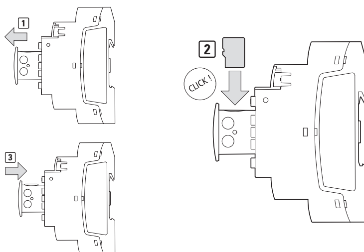
Rys. 29: Umieszczanie karty pamięci
