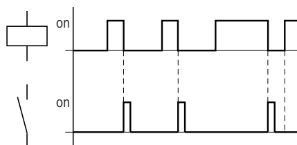
Rys. 96: Wykres działania "Impulsu cyklu" przy opadającym zboczach
