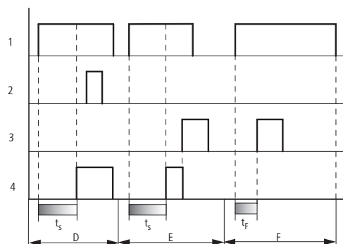
Rys. 139: Wykres działania przekaźnika czasowego o opóźnionym zadziałaniu (z losowym przełączaniem/bez)
