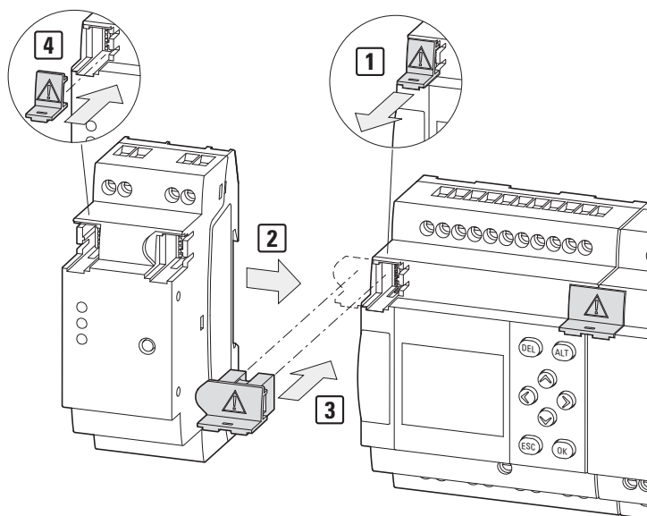
Rys. 6: Montaż urządzenia podstawowego z modułem komunikacyjnym easy jako przykład EASY-COM-SWD-C1
