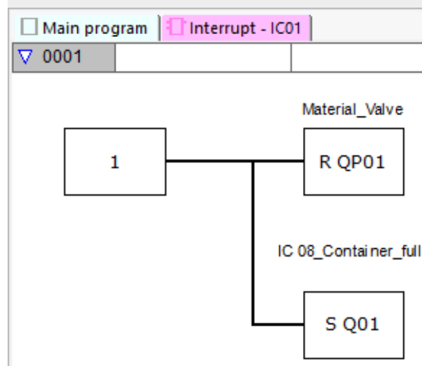
Rys. 253: Program przerwania easySoft 8 - dwa wejścia zliczające
