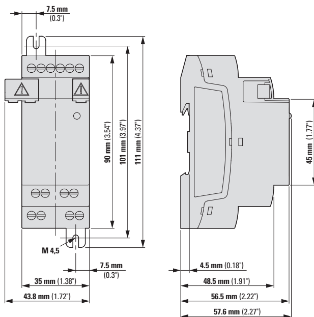
Rys. 360: Wymiary w mm (calach) - rozszerzenia 2TE
