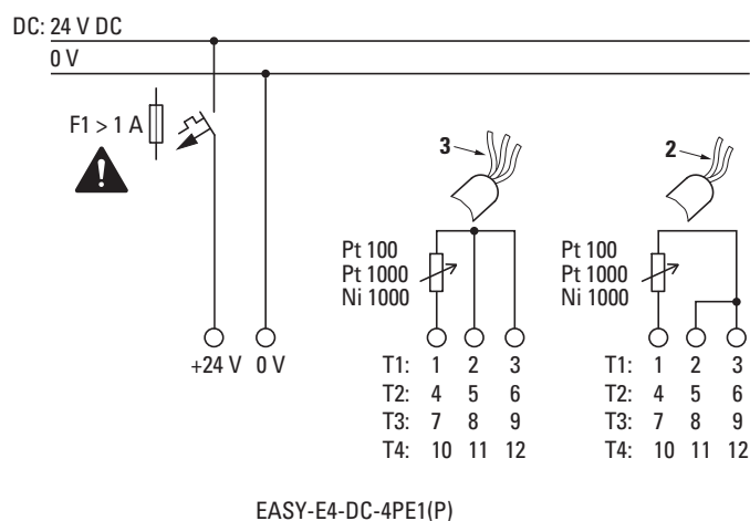
Rys. 25: Podłączanie wejść analogowych EASY-E4-DC-4PE1(P)
