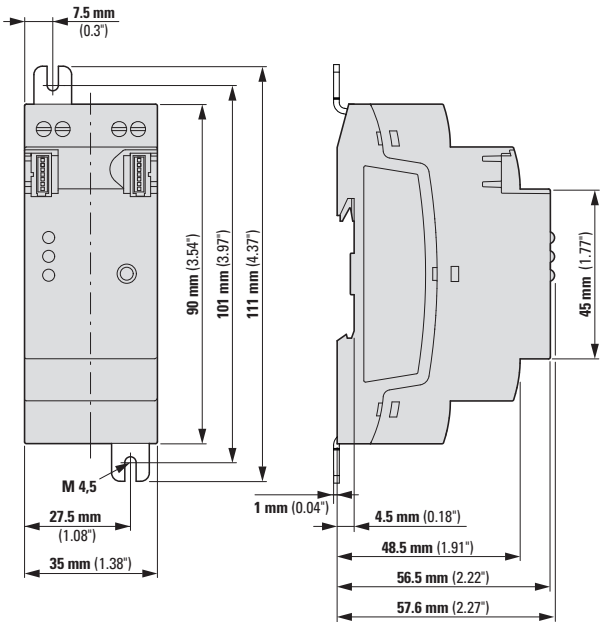
Rys. 362: Wymiary w mm (calach) - rozszerzenia 2TE
