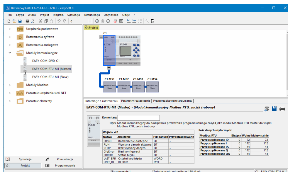
Rys. 342: Pulpit roboczy z urządzeniem podstawowym i modułem komunikacyjnym EASY-COM-RTU-M1 master
