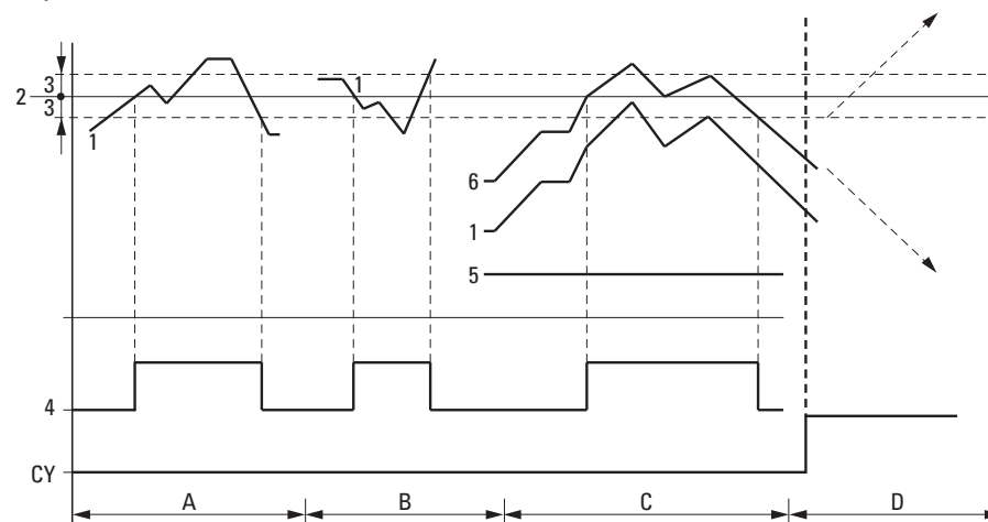
Rys. 171: Wykres działania komparatora wartości analogowych
