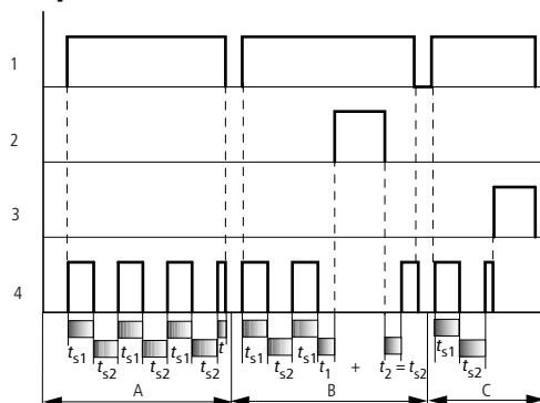
Rys. 145: Wykres działania przełącznika czasowego, formowanie impulsu
