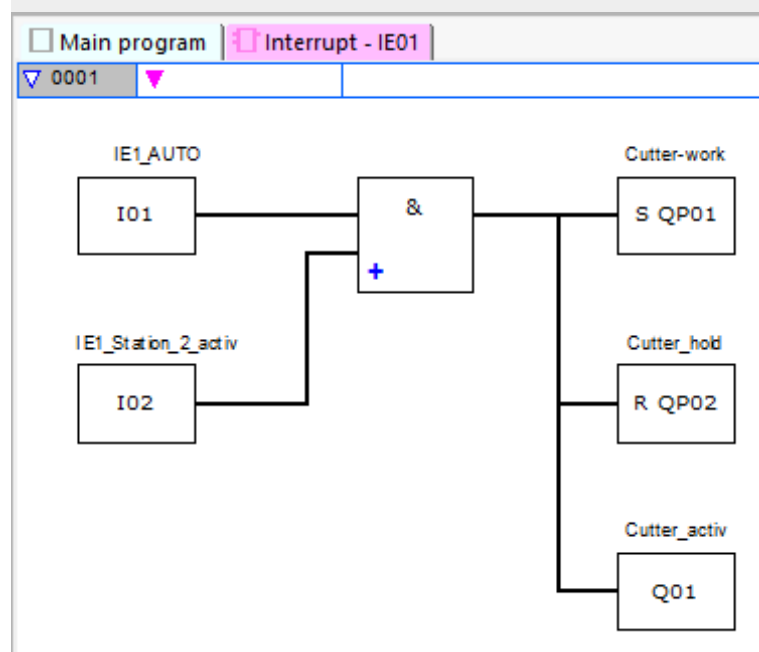
Rys. 260: Program przerwania easySoft 8 - sterowania na podstawie zbocza
