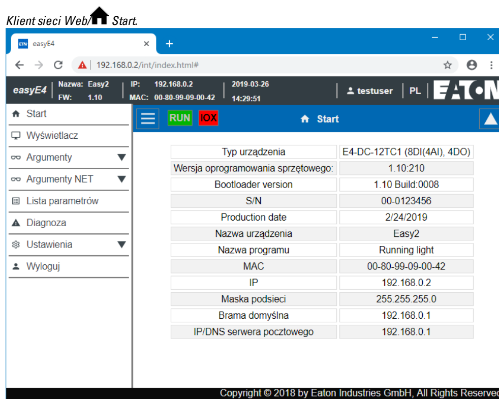
Rys. 315: Klient sieci Web, uruchomiony
