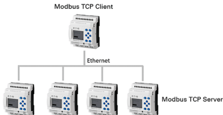
Rys. 344: Jedno urządzenie easyE4 jako klient Modbus TCP steruje czterema serwerami Modbus TCP
