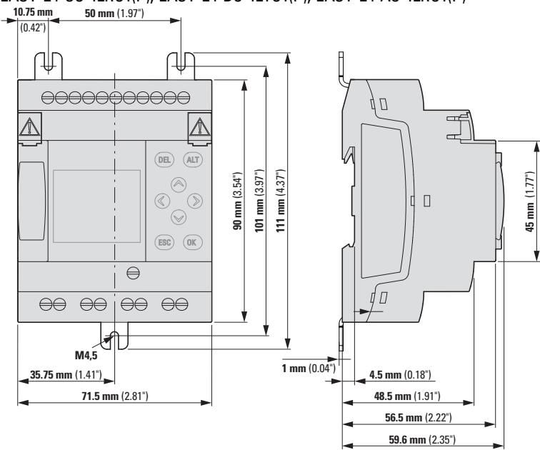
Rys. 357: Wymiary w mm (calach) Urządzenia podstawowe EASY-E4-...-12...C1(P)
