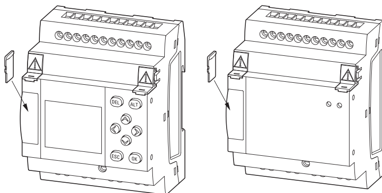
Rys. 27: Gniazdo karty microSD
