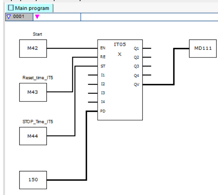
Rys. 262: Program główny easySoft 8 - sterowany czasowo
