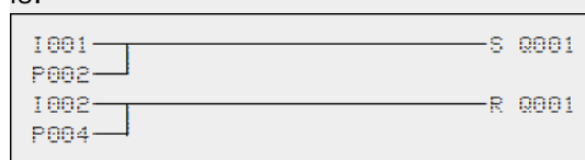
Rys. 107: Przełączanie Q1 za pomocą I1, I2, Í lub za pomocą Ú
