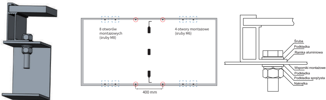
Rysunek 4 Schemat montażu otworu montażowego elementu jednostronnego
