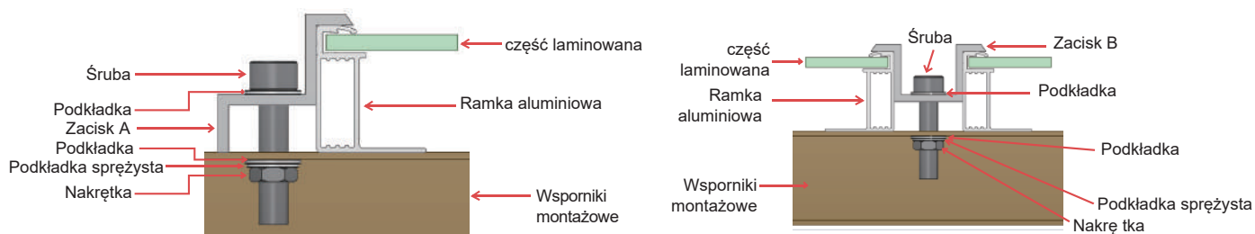
Rysunek 5 Montaż zacisków modułu jednofazowego
