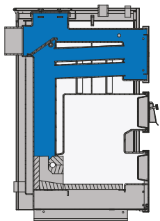
PRZEKRÓJ KOTŁA
