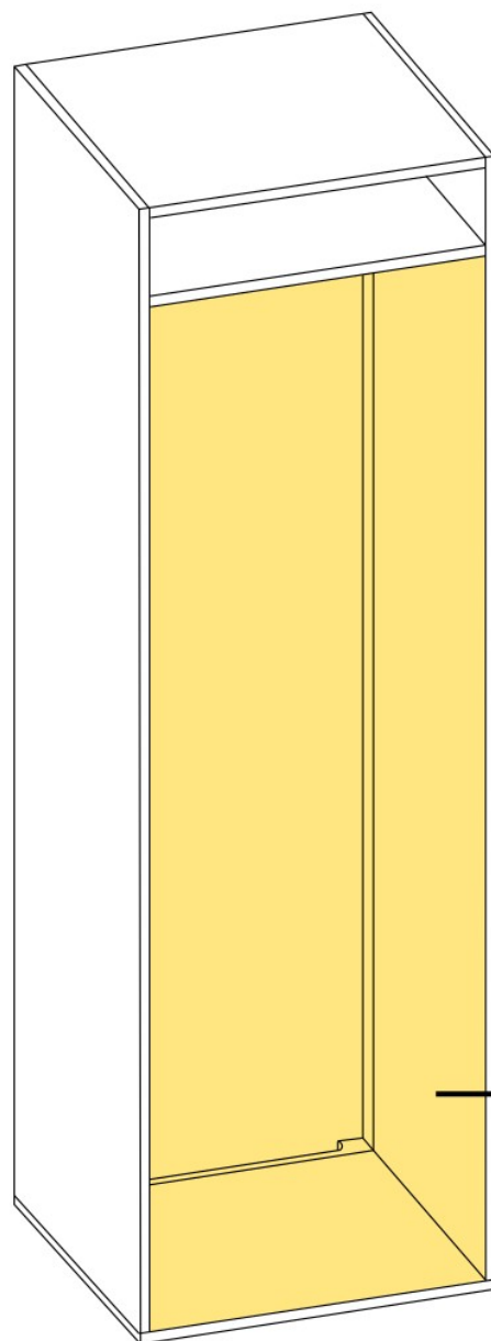
ŁODÓWKA max. 1780/564/565 (szer./wys./gł.)
