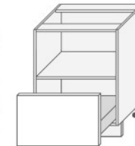
D11K M/60 KOMPAKT ● (600/820/500)
