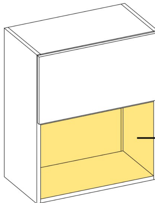
MIKROFALA max. 564/360/305-325* (szer./wys./gł.)
