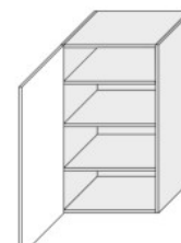
W4 50 (500/960/325)
