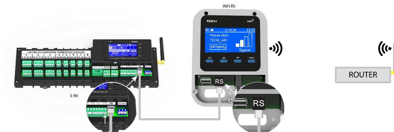
Schemat podpięcia modułu internetowego WiFi RS
