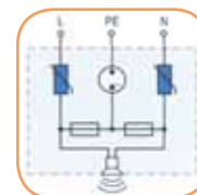
Układ wewnętrzny
