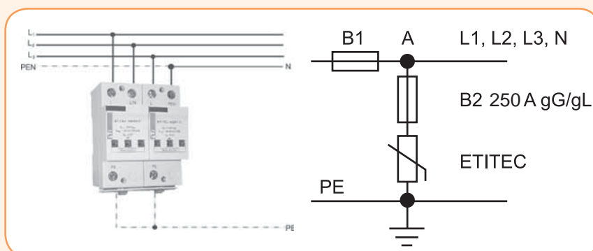
Układ połączeń ogranicznika ETITEC-WENT IT
