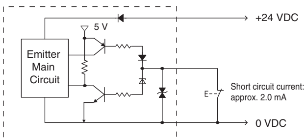
<0 V Inactive>
