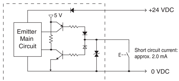
<Short Mode>
