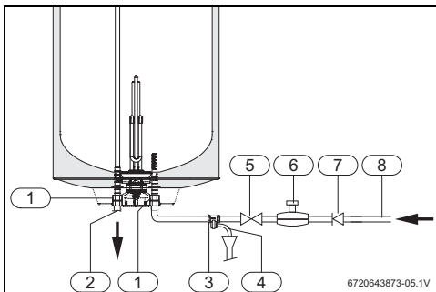
Rys. 8 Przyłącze wody
