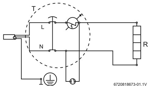
Rys. 4 Schemat połączeń
