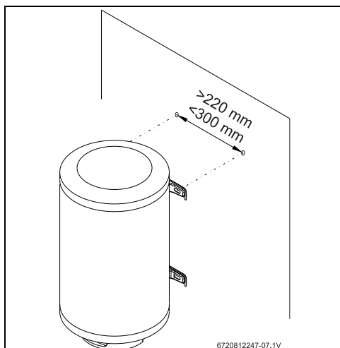
Rys. 6 Montaż pionowy
