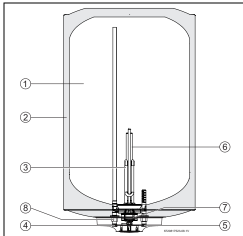
Rys. 3 Konstrukcja podgrzewacza
