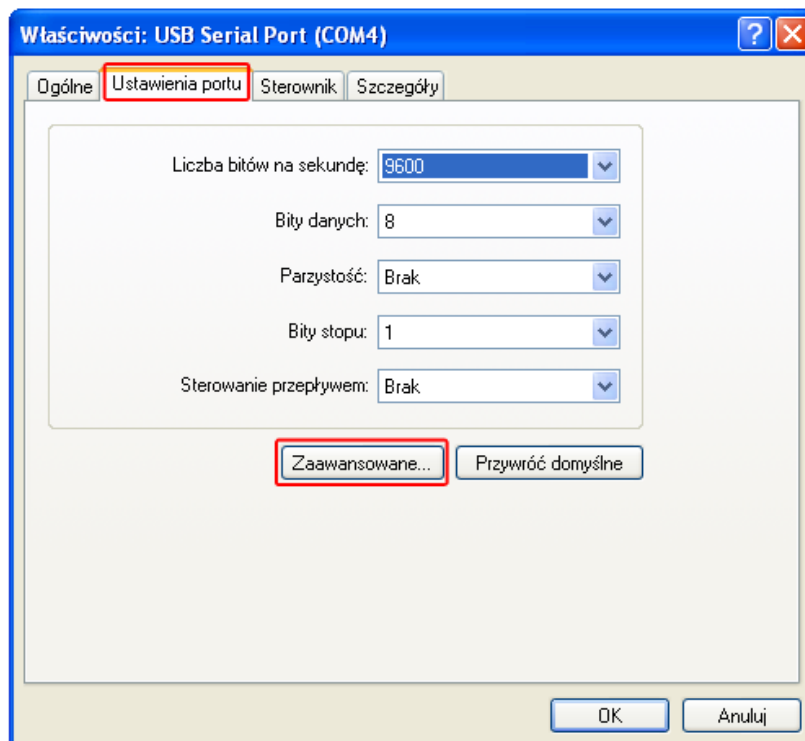
Rysunek 4: Właściwości kontrolera kabla diagnostycznego
