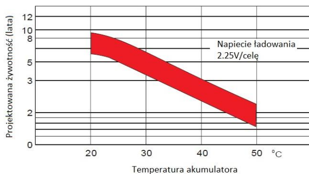
Projektowana żywotność dla pracy buforowej
