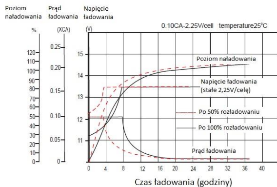
Charakterystyka ładowania - praca buforowa
