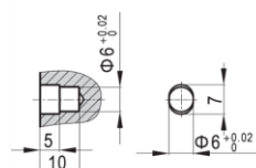
przekrój XX
