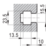
Przekr. rowka T
