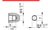
przekrój XX
