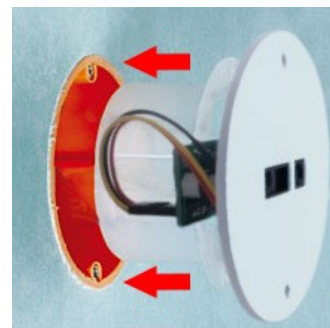
Montaż czujnika ruchu w SesorStep-01 w puszcze fi 60 mm
