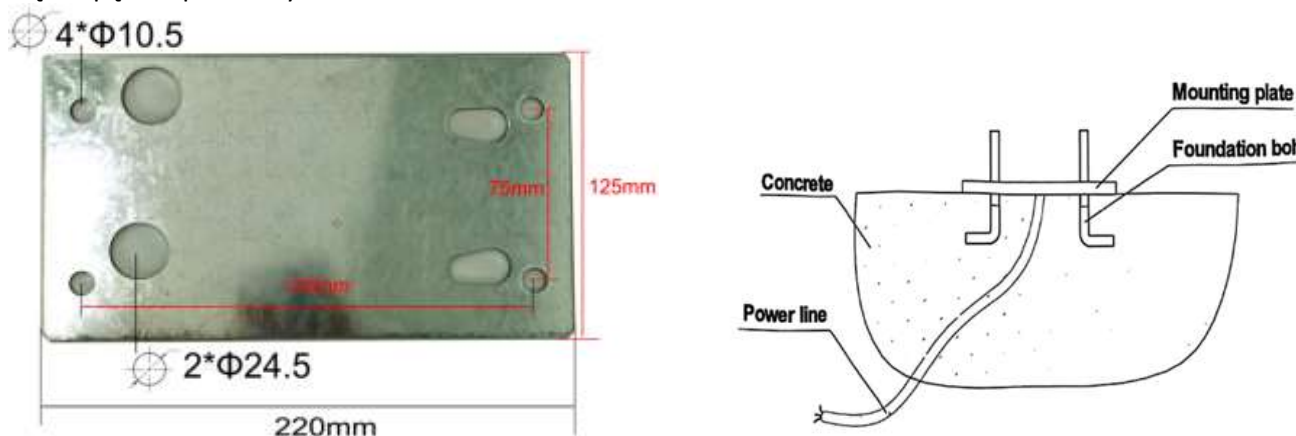
Rys. 2. Sposób montażu napędu na stopie betonowej.
