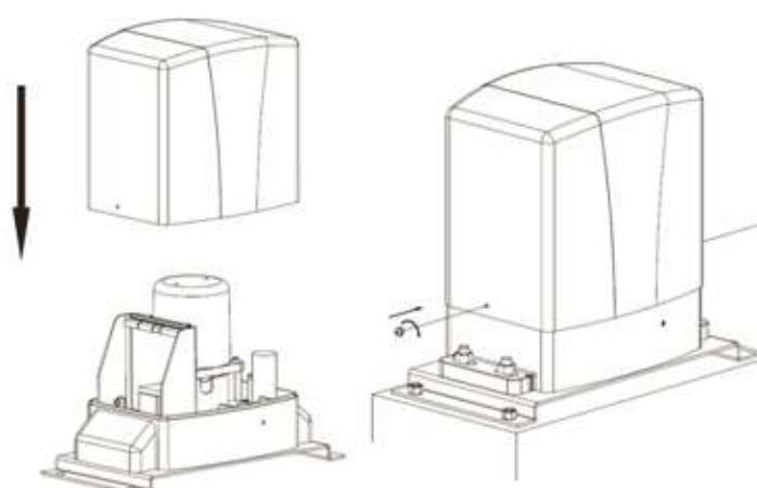
Rys. 6. Instalacja obudowy (rysunki poglądowe)
