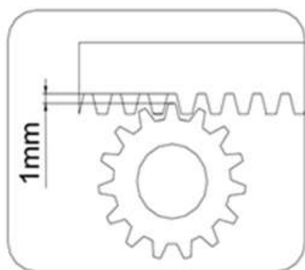
Rys. 3. Dopasowanie koła zębatego do listwy zębatej.
