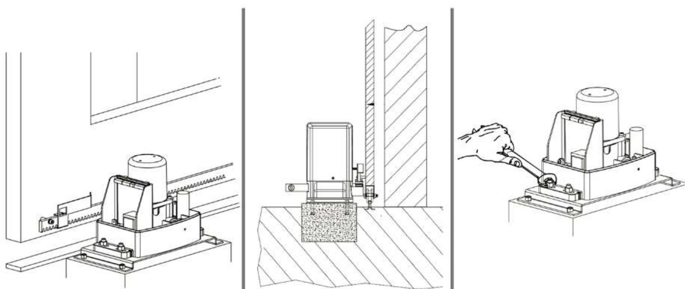
Rys. 5. Położenie napędu względem bramy. (rysunki poglądowe)
